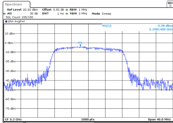
a_5200MHz_Chain 0
