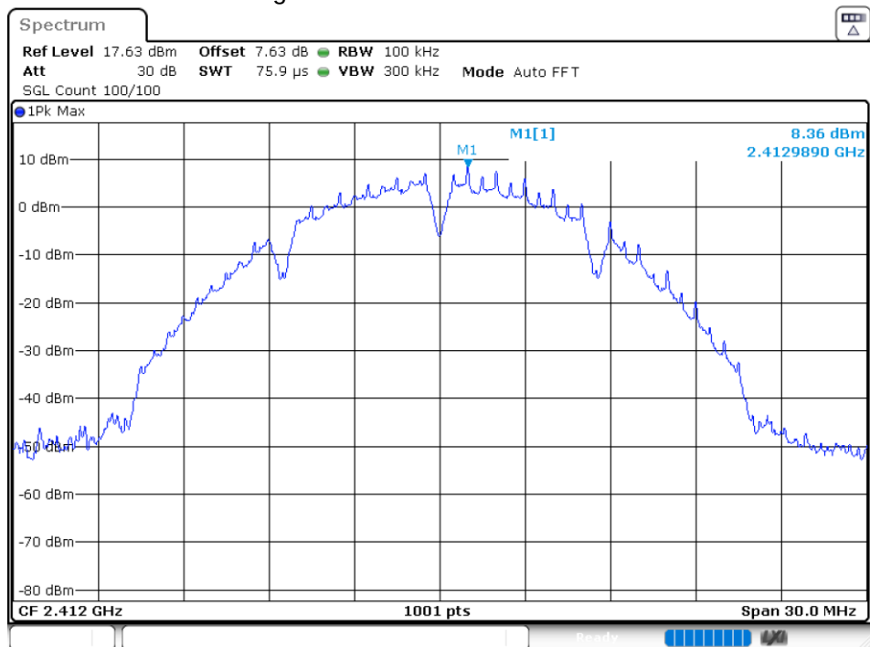
Band Edge NVNT 802.11b 2412MHz Ant 0 Ref
