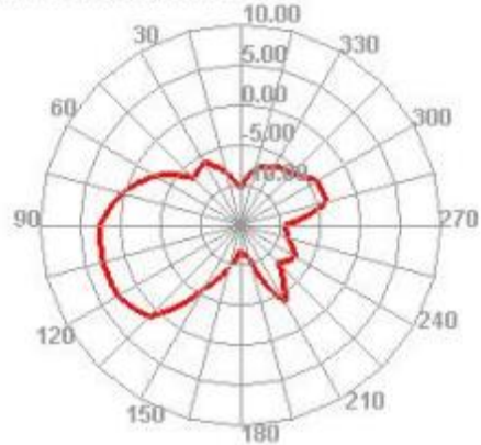
2500.000MHz E2
