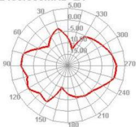
2400.000MHz E1
