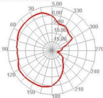
5850.000MHz H
