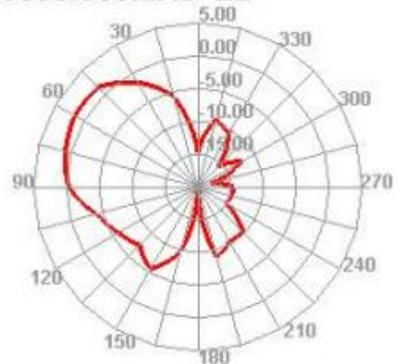
5850.000MHz E2
