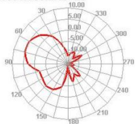
5500.000MHz E2
