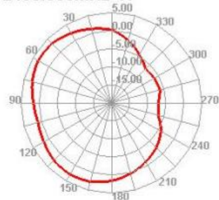
2450.000MHz H
