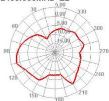
2400.000MHz E2
