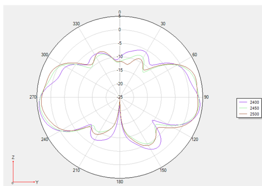
2400MHz\2450MHz\2500MHz YOZ(E2 Face) Gain Icon
