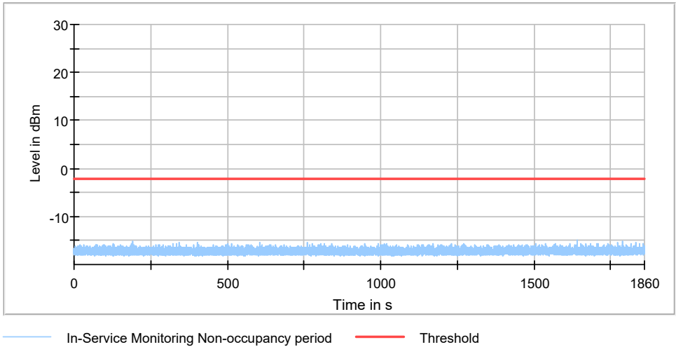
EEE 802.11ac VHT40 5270MHz
