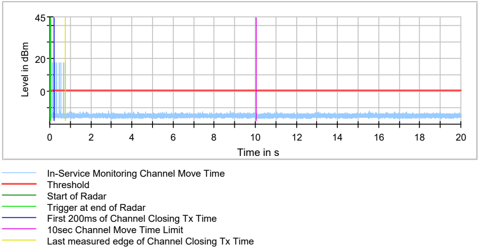
EEE 802.11ac VHT40 5510MHz
