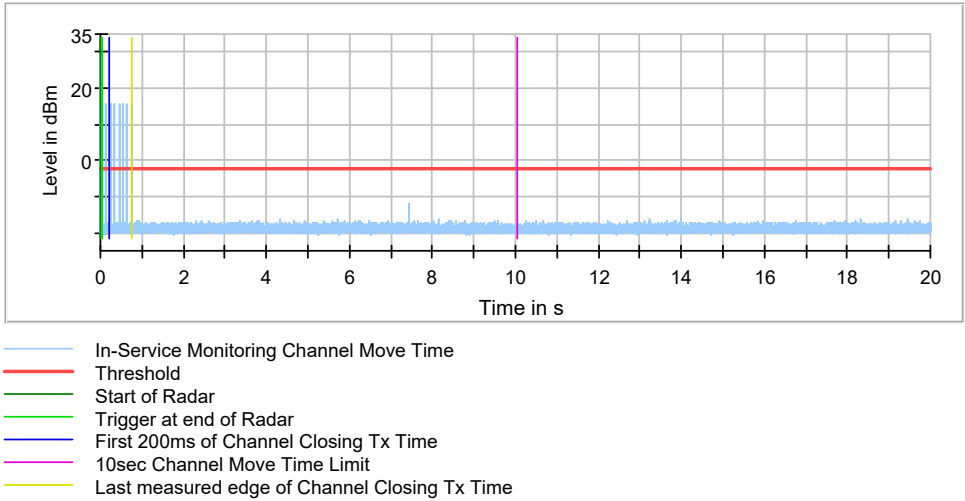
EEE 802.11ac VHT40 5270MHz
