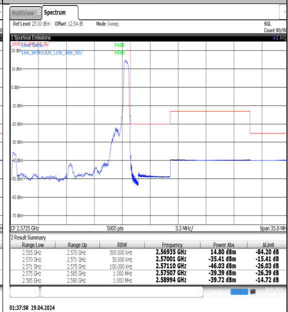
NTNV-N7-PC3-15-15-H-DFT-QPSK- Edge 1RB Right-Ant1-PASS
