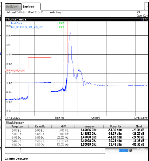
NTNV-N7-PC3-15-40-L-DFT-QPSK- Edge_1RB_Left-Ant1-PASS
