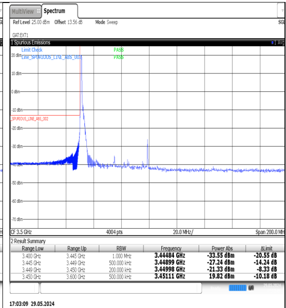
NTNV-N77-3450-3550-PC3-30-50-L-DFT-QPSK- Edge_1RB_Left-Ant1-PASS
