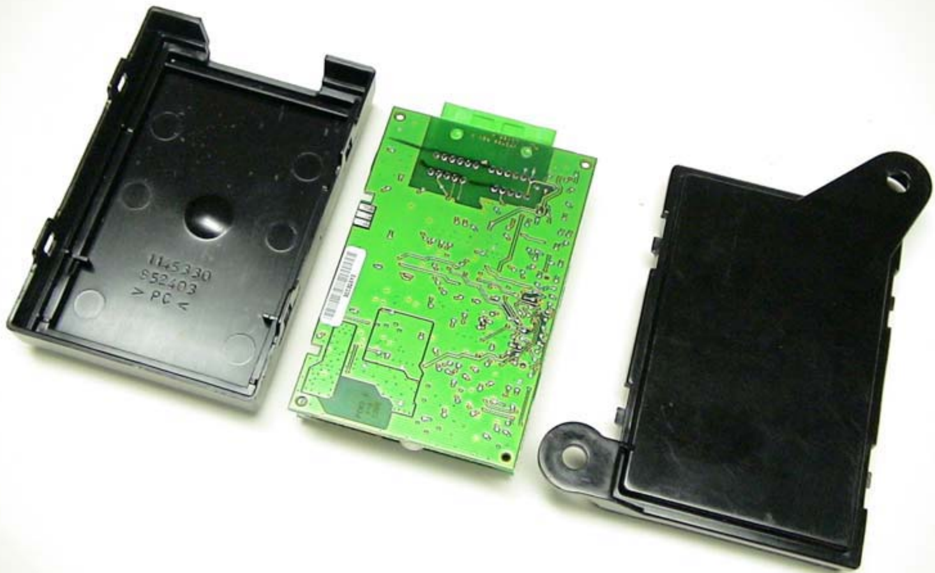
DUT apart (bottom)
