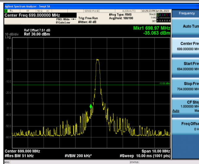
Band12-3MHz-QPSK-23025-1-0-Low--35.06-PASS
