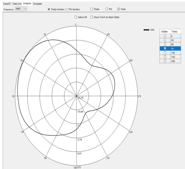
2400MHz
