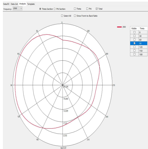
2500MHz
