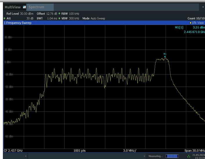
11BE20MIMO_Ant0_2437_26Tone_RU8_0~Reference
