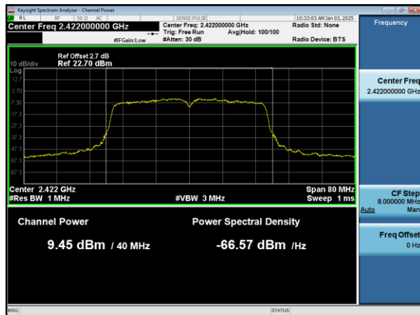
802.11n(HT40) ANT 1
