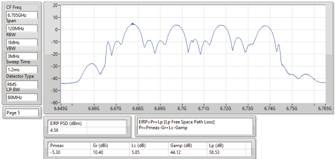
EIRP PSD;Band:6.7G;be80;BWch:80MHz;Nss:1,(M0);Nant:4;Ch:6705MHz;TX
