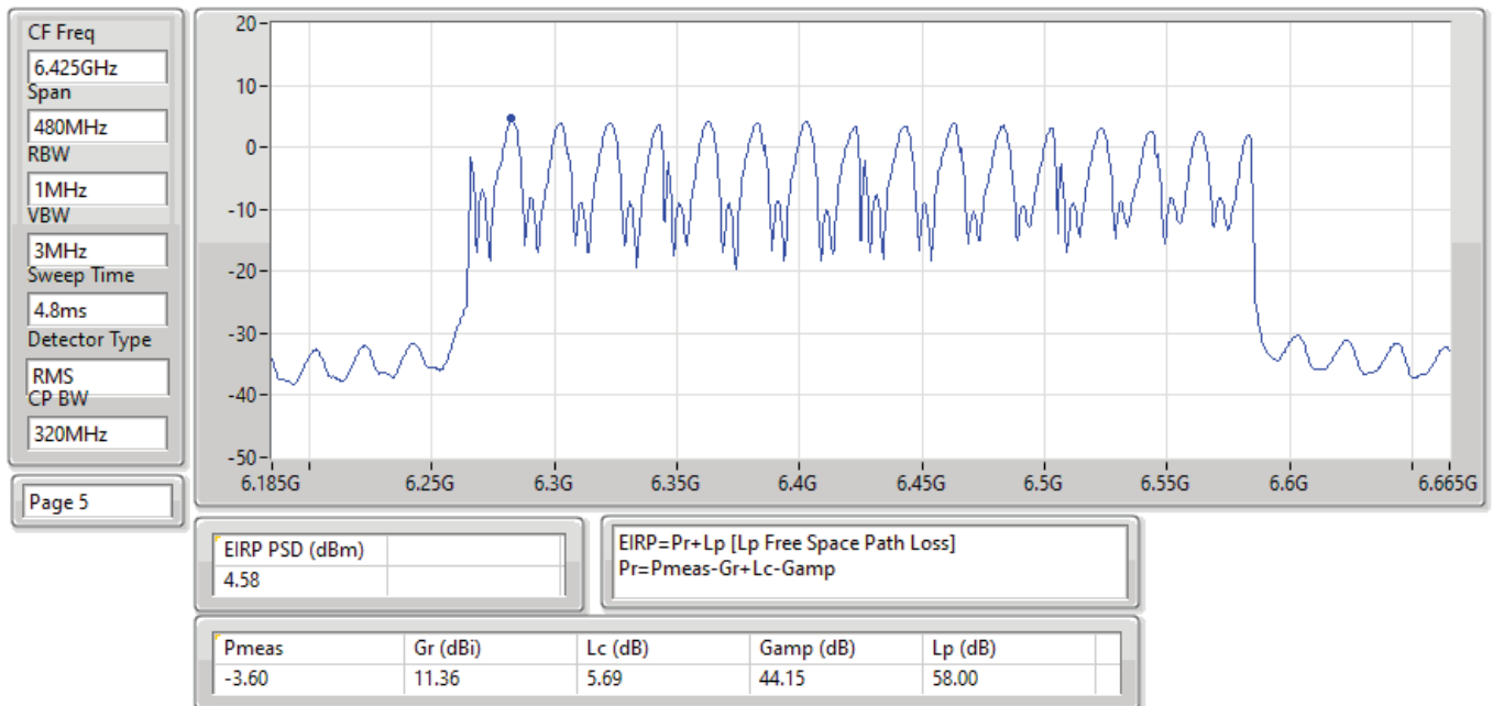
EIRP PSD;Band:6.2G;be320;BWch:320MHz;Nss:1,(M0);Nant:4;Ch:6425MHz;TX
