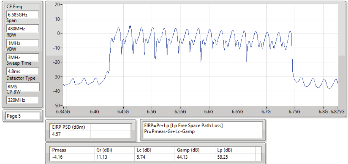
EIRP PSD;Band:6.4G;be320;BWch:320MHz;Nss:1,(M0);Nant:4;Ch:6585MHz;TX
