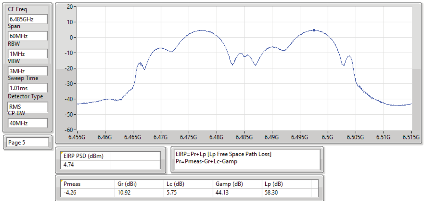
EIRP PSD;Band:6.4G;be40;BWch:40MHz;Nss:1,(M0);Nant:4;Ch:6485MHz;TX
