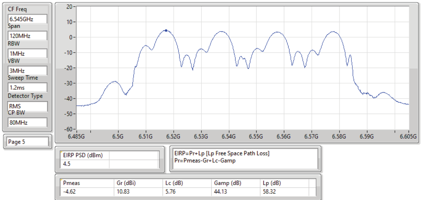
EIRP PSD;Band:6.4G;be80;BWch:80MHz;Nss:1,(M0);Nant:4;Ch:6545MHz;TX
