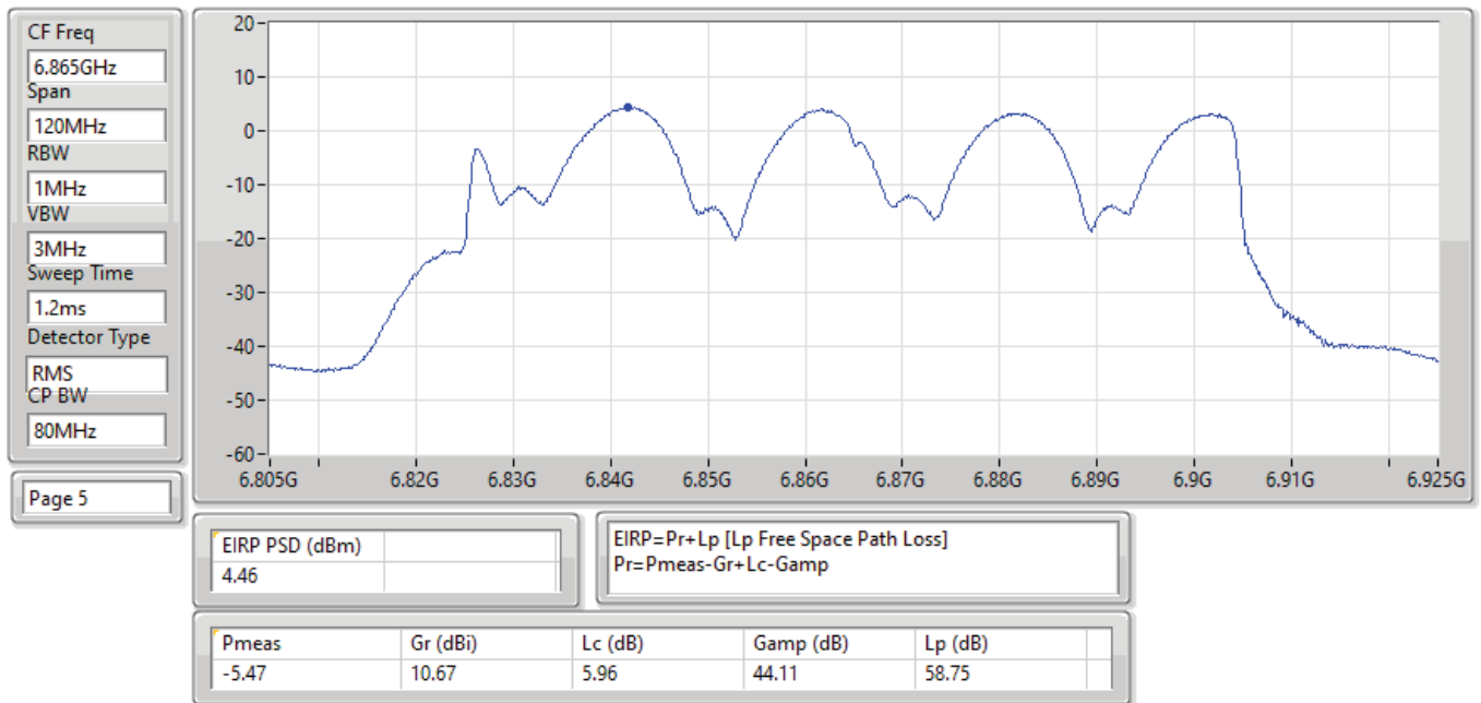
EIRP PSD;Band:6.7G;be80;BWch:80MHz;Nss:1,(M0);Nant:4;Ch:6865MHz;TX
