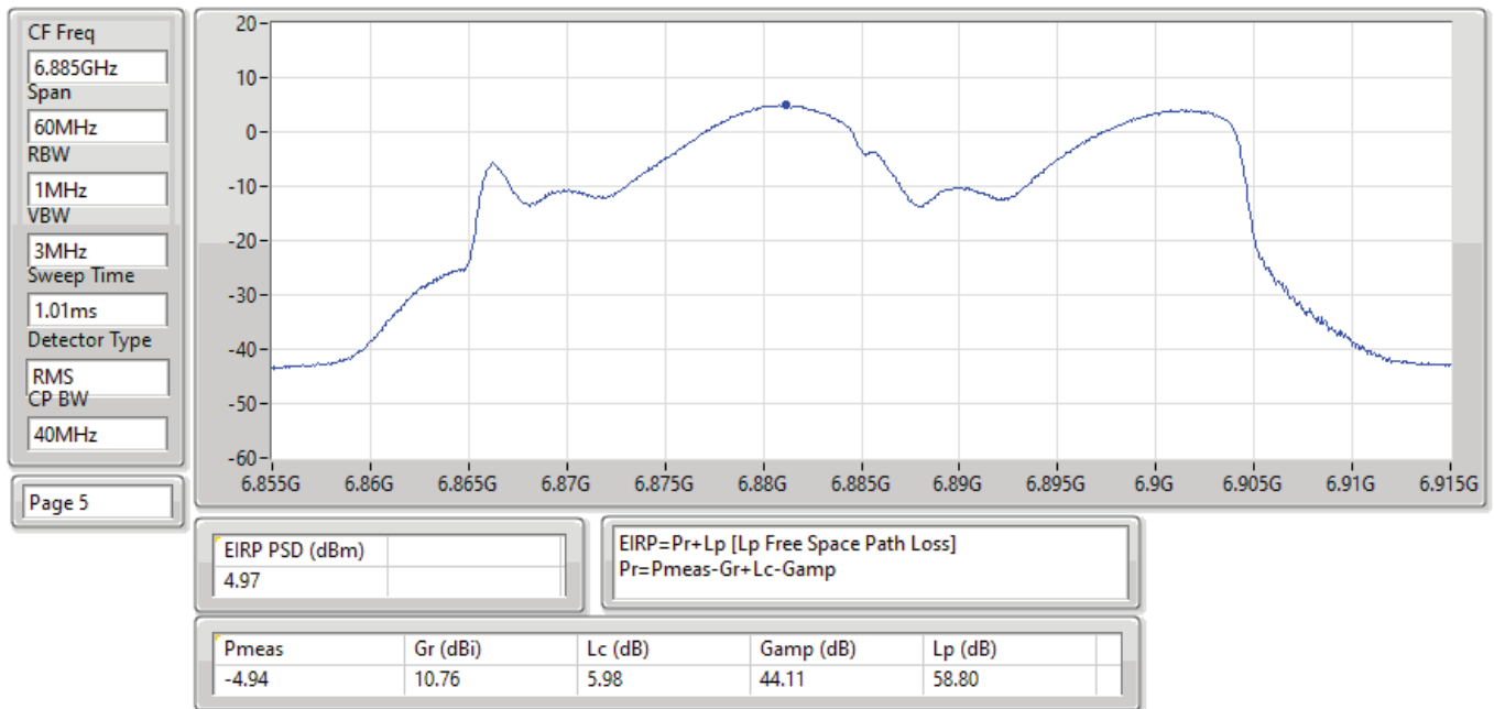
EIRP PSD;Band:6.7G;be40;BWch:40MHz;Nss:1,(M0);Nant:4;Ch:6885MHz;TX
