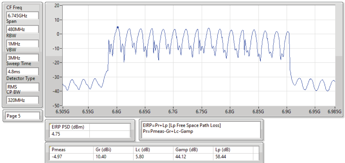
EIRP PSD;Band:6.7G;be320;BWch:320MHz;Nss:1,(M0);Nant:4;Ch:6745MHz;TX
