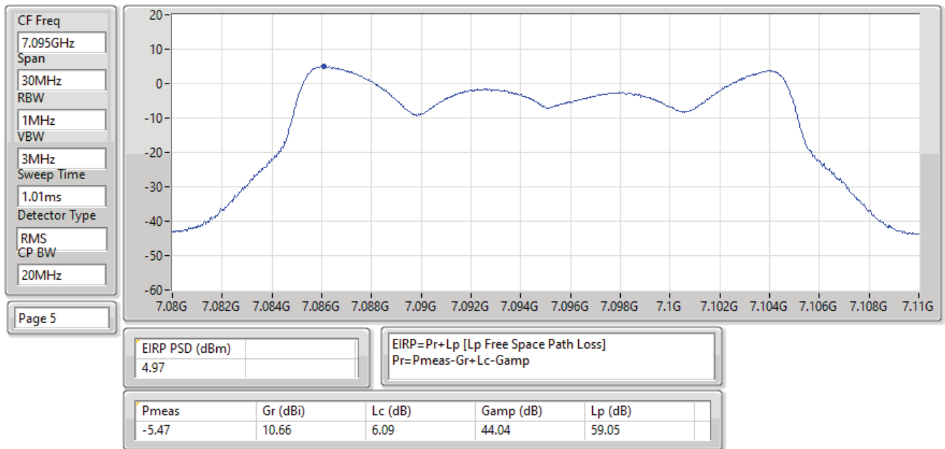
EIRP PSD;Band:7.0G;be20;BWch:20MHz;Nss:1,(M0);Nant:4;Ch:7095MHz;TX
