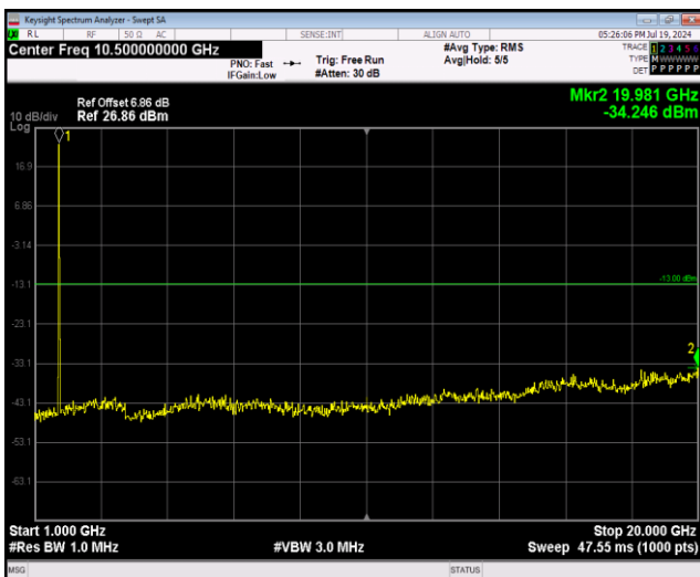
Band66-20MHz-QPSK-132322-1RB#0-Range2:1000~20000MHz
