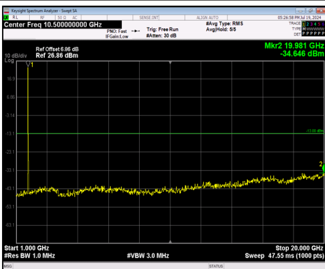
Band66-20MHz-QPSK-132572-1RB#0-Range2:1000~20000MHz
