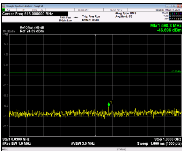
Band66-20MHz-QPSK-132572-1RB#0-Range1:30~1000MHz
