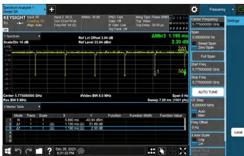
NTVN-11AC80MIMO-Ant0-5775
