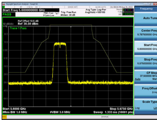
U-NII-3 ,Plot 1,Band Edge-802.11ax(40 MHz),5795MHz,Ant0
