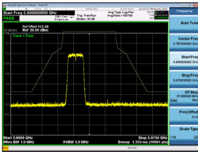
U-NII-3 ,Plot 1,Band Edge-802.11ac(40 MHz),5795MHz,Ant0
