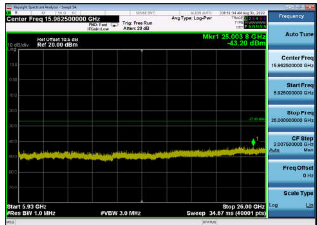
U-NII-3 ,Plot 3,5925MHz~26000MHz-802. 11n(20MHz),5825MHz,Ant1
