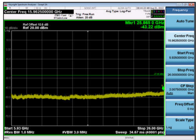
U-NII-3 ,Plot 3,5925MHz~26000MHz-802. 11n(20MHz),5825MHz,Ant1
