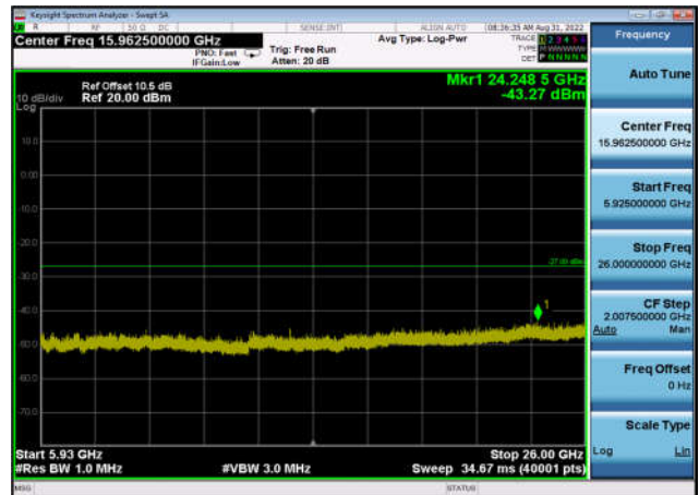
U-NII-3 ,Plot 3,5925MHz~26000MHz-802. 11n(20MHz),5785MHz,Ant1
