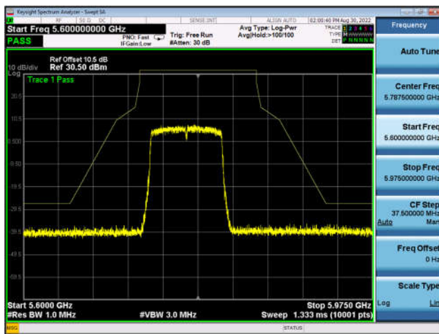
U-NII-3 ,Plot 1,Band Edge-802.11ac(80 MHz),5775MHz,Ant0
