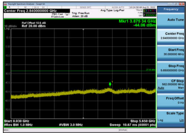
U-NII-3 ,Plot 2,30MHz~5650MHz-802.11a x(20MHz),5785MHz,Ant1
