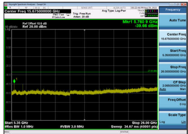
U-NII-1 ,Plot 3,5350MHz~26000MHz-802. 11ac(20MHz),5240MHz,Ant1
