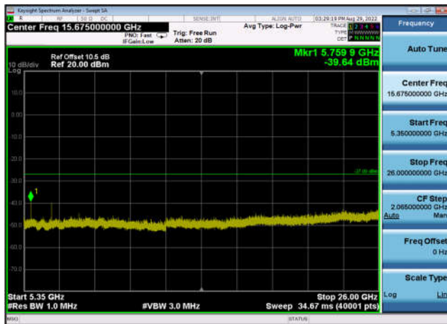
U-NII-1 ,Plot 3,5350MHz~26000MHz-802. 11ax(80MHz),5210MHz,Ant0
