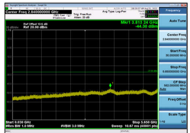
U-NII-3 ,Plot 2,30MHz~5650MHz-802.11n (40MHz),5755MHz,Ant1
