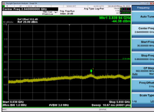
U-NII-3 ,Plot 2,30MHz~5650MHz-802.11n (20MHz),5785MHz,Ant0
