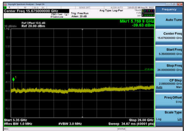
U-NII-1 ,Plot 3,5350MHz~26000MHz-802. 11ax(80MHz),5210MHz,Ant1
