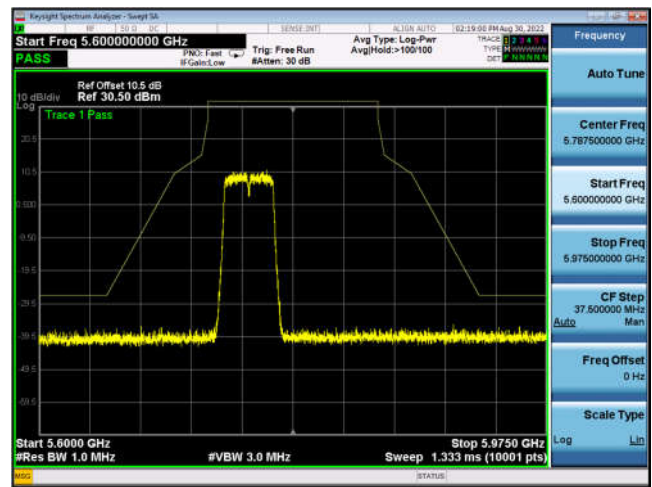
U-NII-3 ,Plot 1,Band Edge-802.11ac(40 MHz),5795MHz,Ant1
