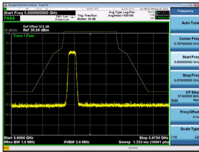
U-NII-3 ,Plot 1,Band Edge-802.11n(20 Hz),5785MHz,Ant0
