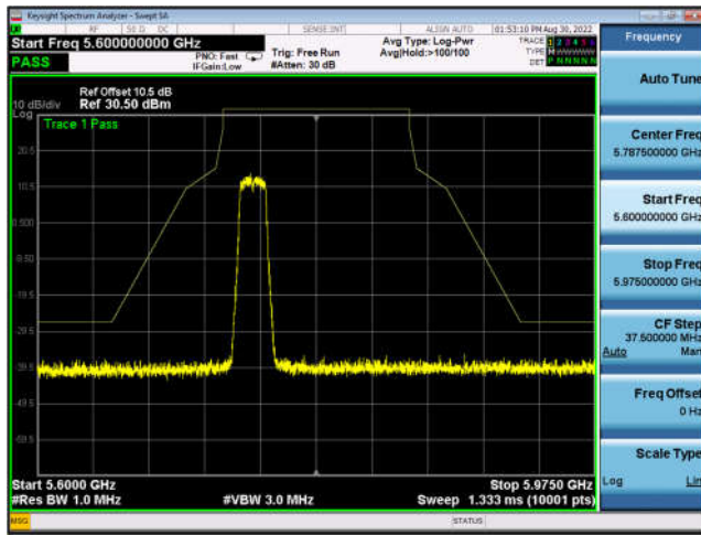
U-NII-3 ,Plot 1,Band Edge-802.11ac(20 MHz),5785MHz,Ant0
