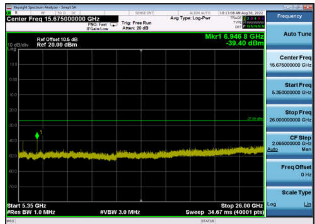
U-NII-1 ,Plot 3,5350MHz~26000MHz-802. 11ax(80MHz),5210MHz,Ant1
