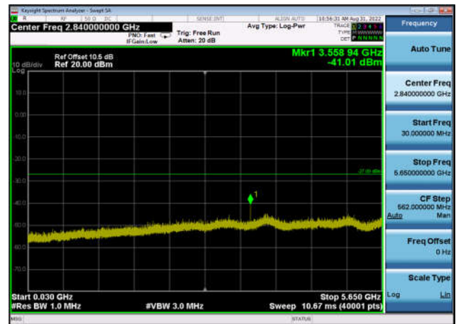
U-NII-3 ,Plot 2,30MHz~5650MHz-802.11a x(80MHz),5775MHz,Ant1
