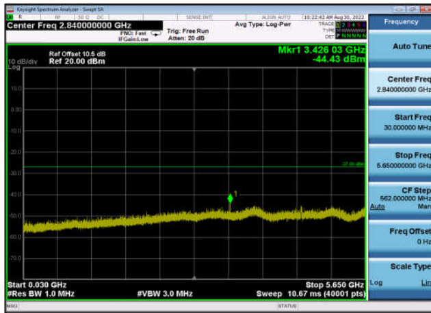
U-NII-3 ,Plot 2,30MHz~5650MHz-802.11a (20MHz),5785MHz,Ant0
