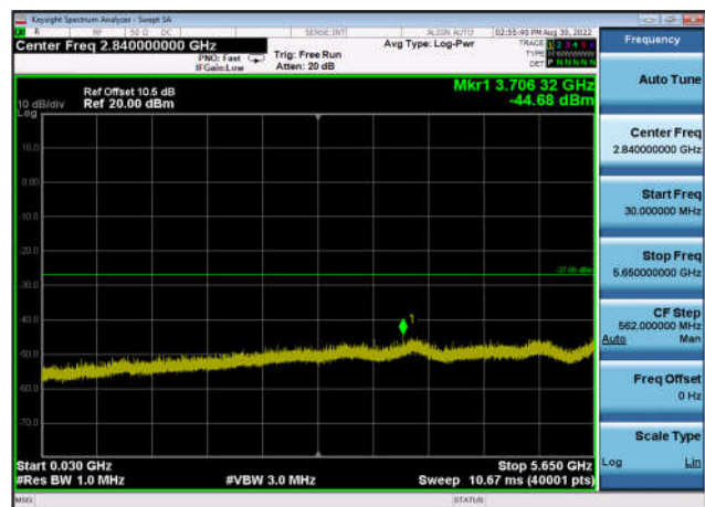
U-NII-3 ,Plot 2,30MHz~5650MHz-802.11n (40MHz),5755MHz,Ant0
