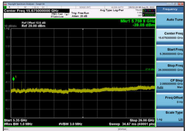
U-NII-1 ,Plot 3,5350MHz~26000MHz-802. 11ax(40MHz),5230MHz,Ant1
