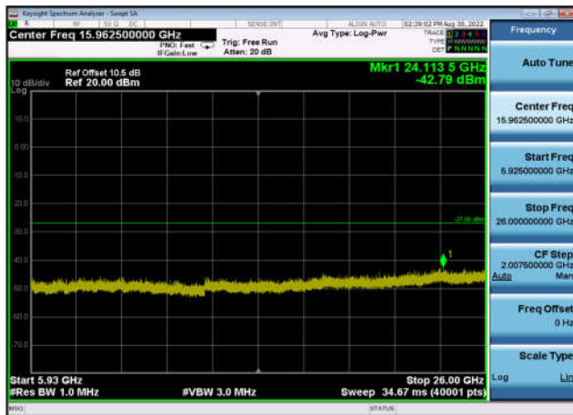
U-NII-3 ,Plot 3,5925MHz~26000MHz-802. 11n(20MHz),5825MHz,Ant0
