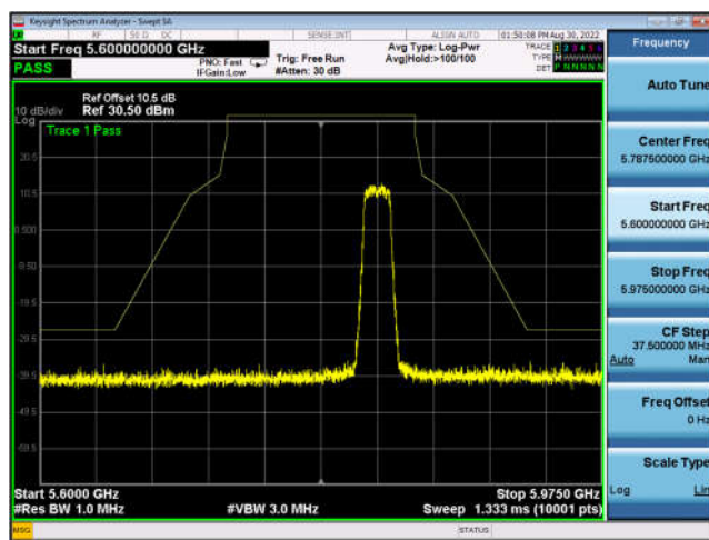
U-NII-3 ,Plot 1,Band Edge-802.11n(20 Hz),5825MHz,Ant0
