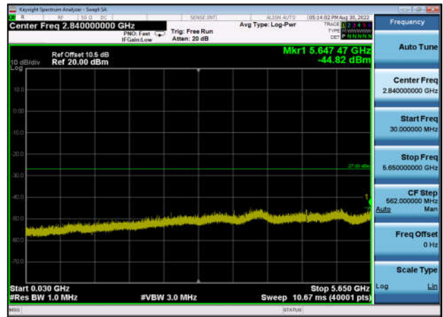
U-NII-3 ,Plot 2,30MHz~5650MHz-802.11a (20MHz),5785MHz,Ant1
