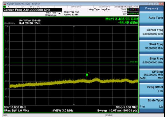
U-NII-3 ,Plot 2,30MHz~5650MHz-802.11a x(20MHz),5825MHz,Ant1
