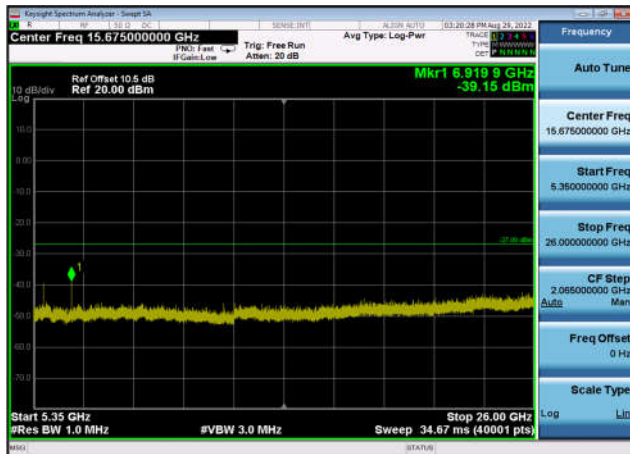
U-NII-1 ,Plot 3,5350MHz~26000MHz-802. 11ax(40MHz),5230MHz,Ant0
