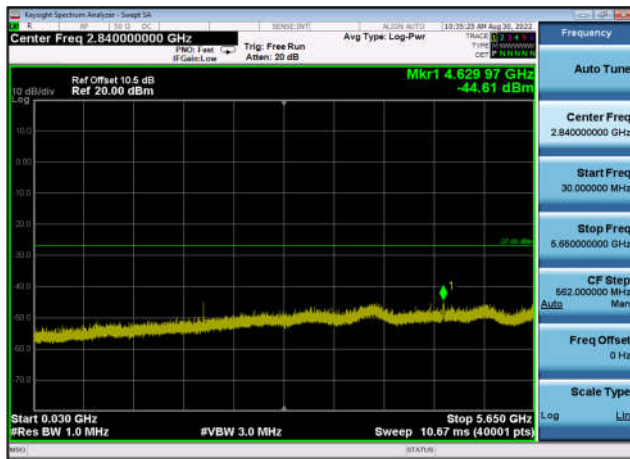
U-NII-3 ,Plot 2,30MHz~5650MHz-802.11a (20MHz),5825MHz,Ant0
