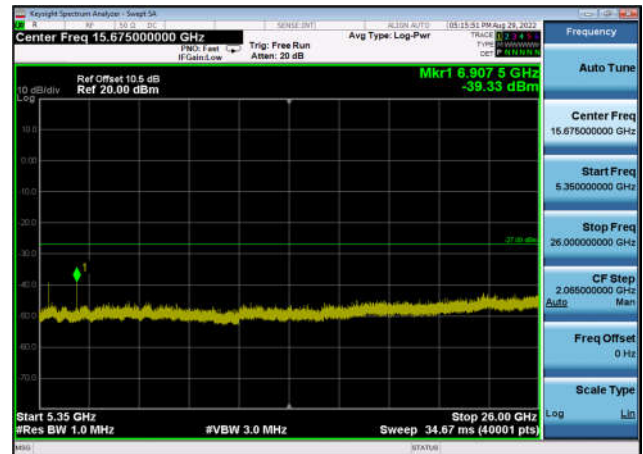
U-NII-1 ,Plot 3,5350MHz~26000MHz-802. 11ac(20MHz),5220MHz,Ant1
