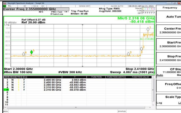
3DH5_Ant1_Low_Hop_2402
