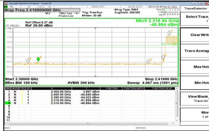
DH5_Ant1_Low_Hop_2402
