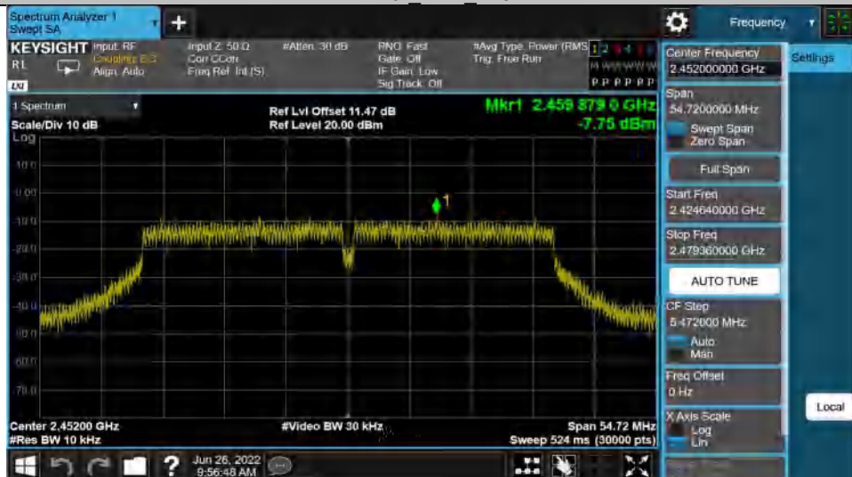
11N40- Ant1 2452
