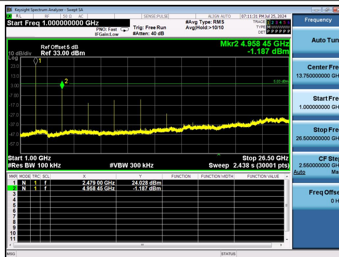
2.4G-Ant1-2479.4-1000~26500-PASS
