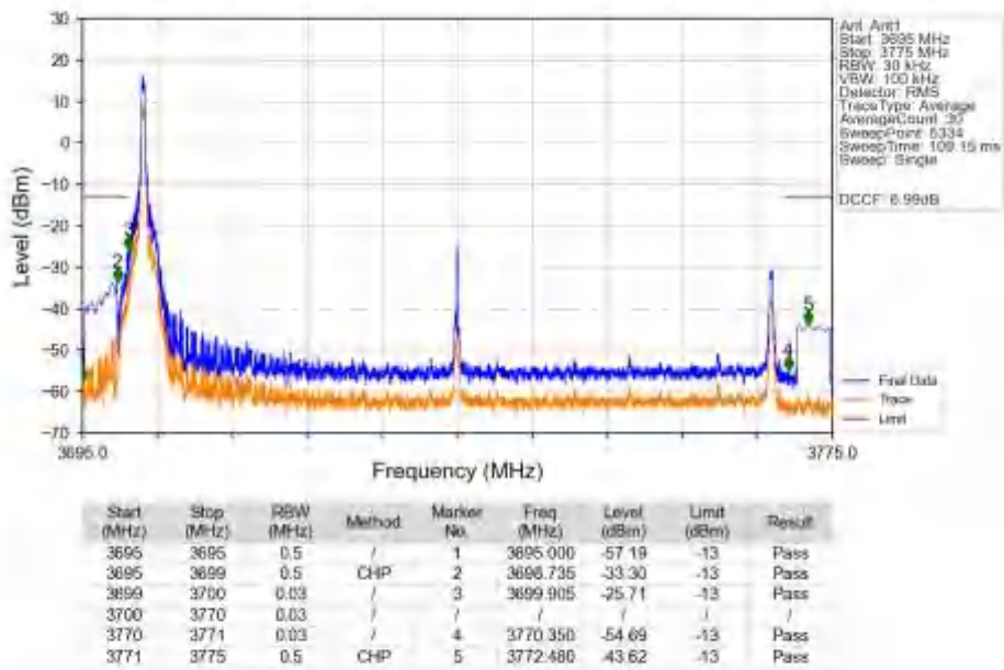
n77a_30kHz_SISO_NTNV_70MHz_CP-OFDM_QPSK_3735MHz_Inner_1RB_Left_Ant1
