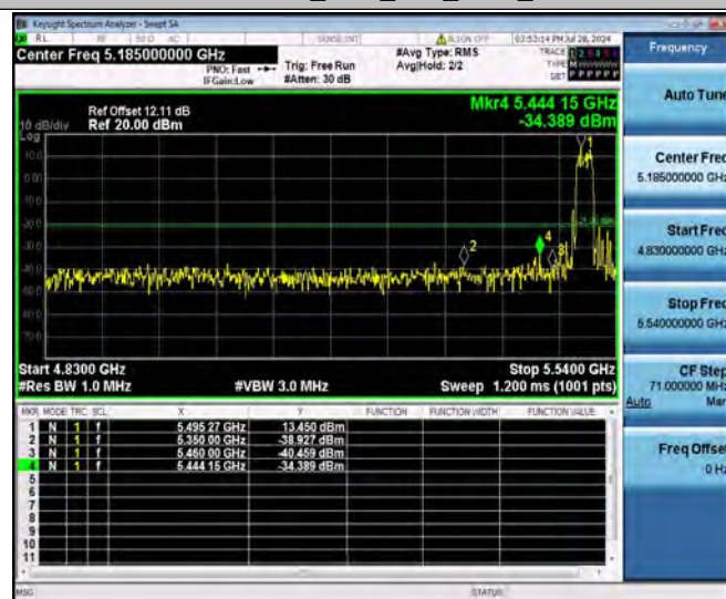
11AX40SISO_Ant1_Low_5510_AV
