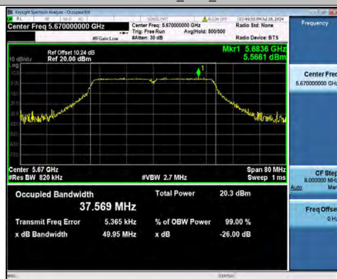
11AX20SISO_Ant1_5500
