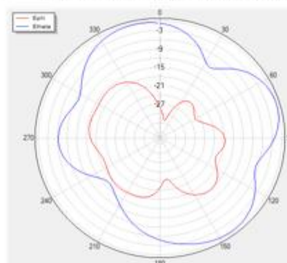
Theta=90 freq=1600MHz
