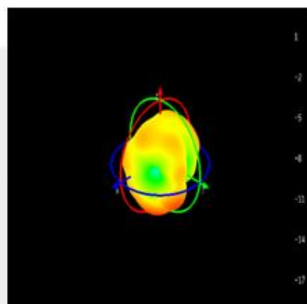
Theta=90 freq=1600MHz
