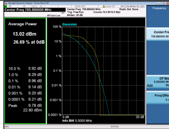
B12-5M-Mid CH-PAPR-QPSK
