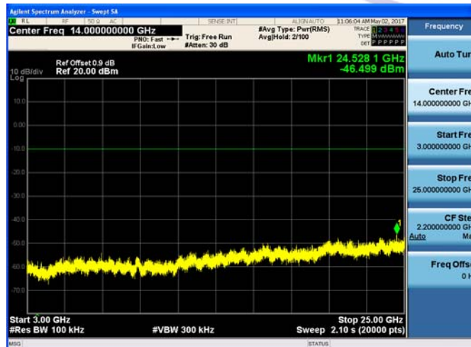
3GHz-25GHz
