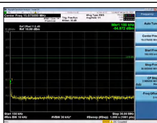
Band26(824-849)-3MHz-QPSK-26915-1RB#0-0. 15~30-PASS
