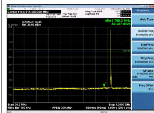
Band26(824-849)-3MHz-QPSK-26915-1RB#0-30 ~1000-PASS
