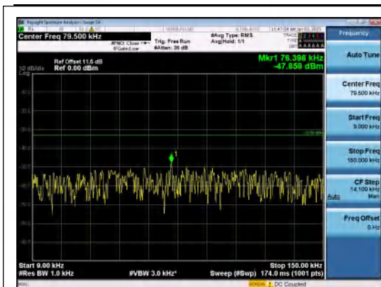
Band26(824-849)-3MHz-QPSK-26915-1RB#0-0. 009~0.15-PASS
