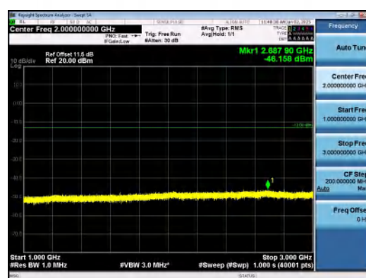
Band26(824-849)-3MHz-QPSK-26915-1RB#0-10 00~3000-PASS
