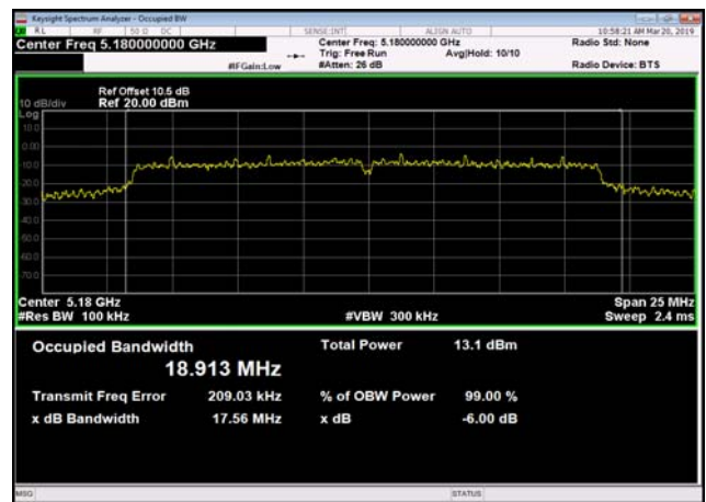
U-NII-1 6dB Bandwidth-802.11ac(20MHz) ,5180MHz,Ant1
