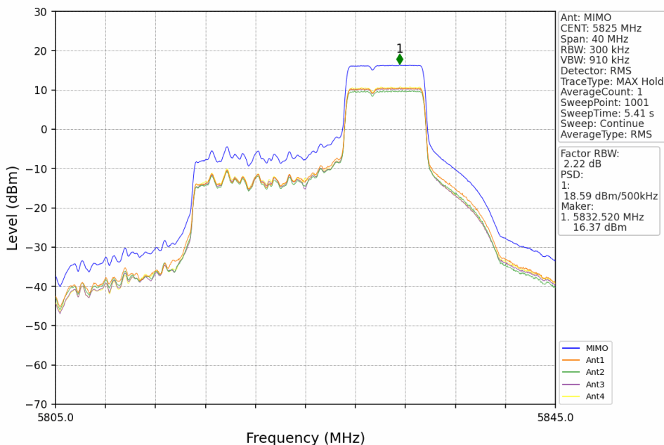
802.11be(EHT20)_HCH_5825MHz_RU52_Right_MIMO_NTNV
