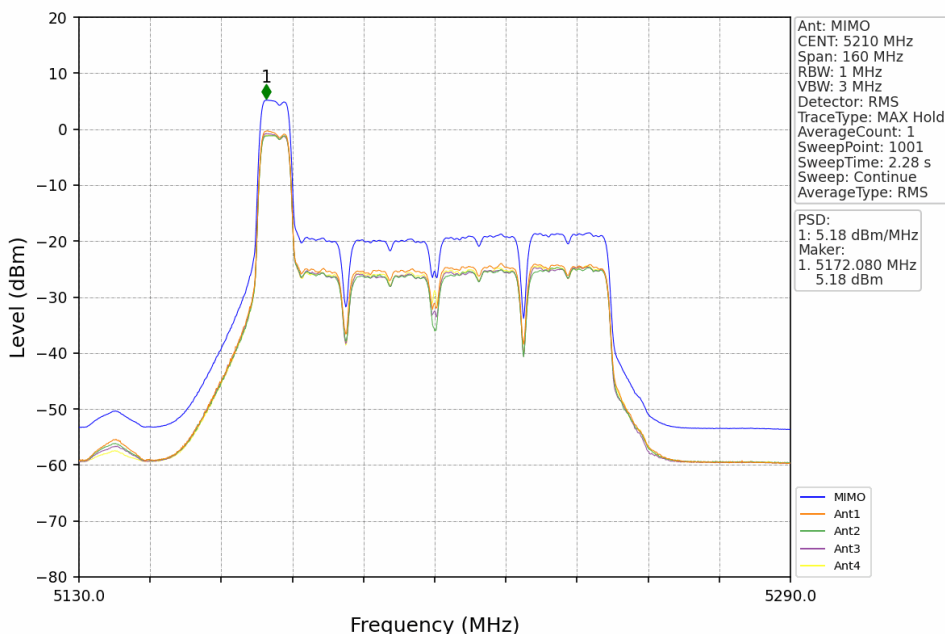
802.11be(EHT80)_MCH_5210MHz_RU996_Left_MIMO_NTNV
