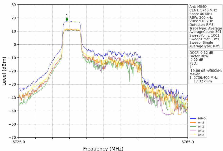
802.11be(EHT20)_LCH_5745MHz_RU52_Left_MIMO_NTNV
