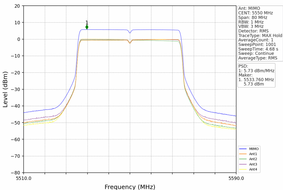
802.11be(EHT40)_MCH_5550MHz_RU484_Left_MIMO_NTNV
