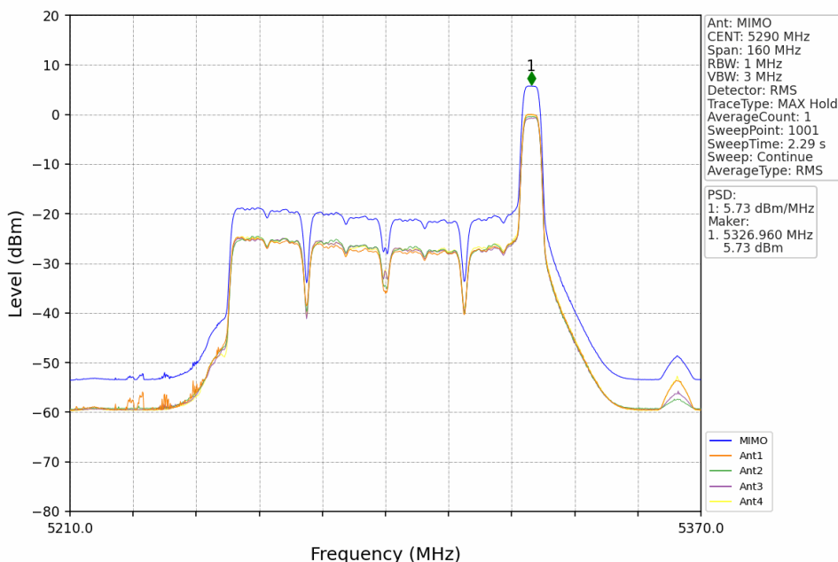
802.11be(EHT80)_MCH_5290MHz_RU52+26_Right_MIMO_NTNV
