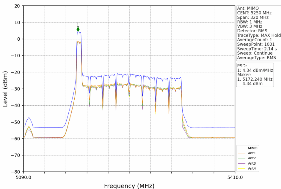
802.11be(EHT160)_MCH_5250MHz_RU52+26_Left_MIMO_NTNV
