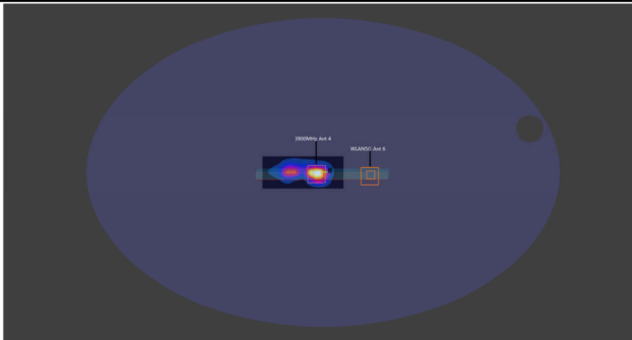
WWAN+ WLAN 5GHz Ant6+NFC_ Edge 3 0mm
