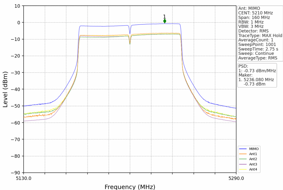
802.11ac(VHT80)_MCH_5210MHz_MIMO_NTNV
