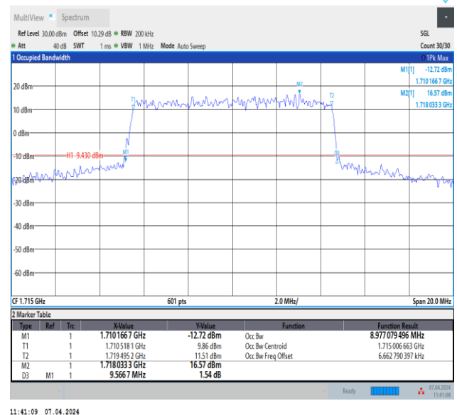
Band4-10MHz-QPSK-20000-50RB#0-PASS
