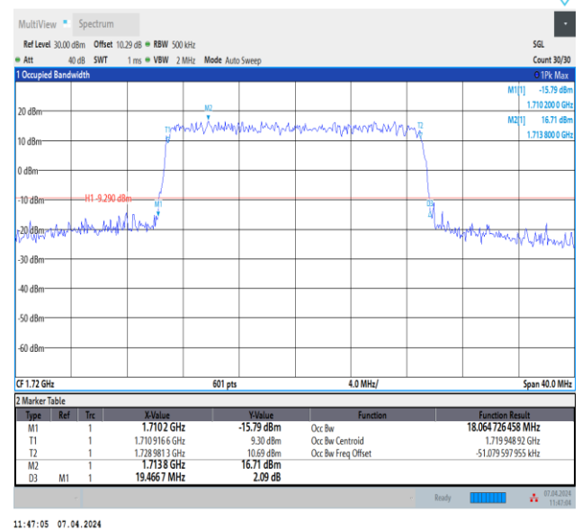
Band4-20MHz-QPSK-20050-100RB#0-PASS
