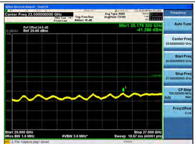
Band41-20G-27G / 10MHz / Low CH / QPSK
