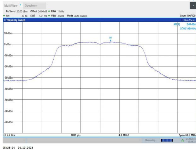
11AC20MIMO_Ant2_5700
