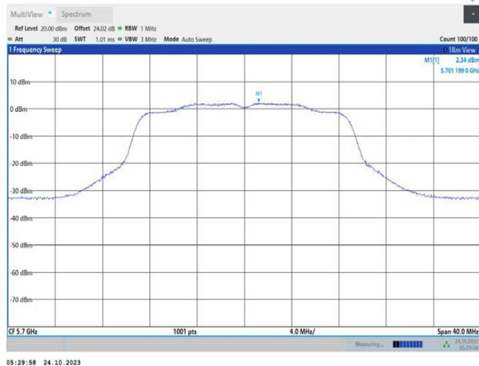
11AC20MIMO_Ant2_5700
