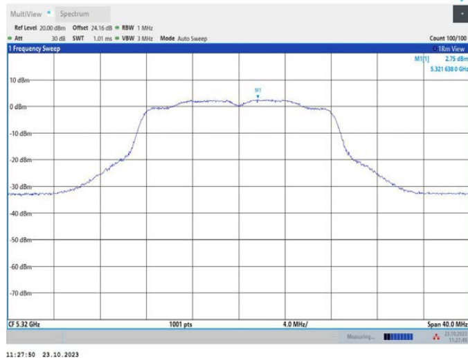
11A_Ant2_5320
