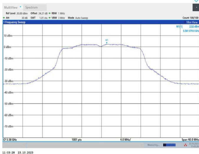
11A_Ant1_5580
