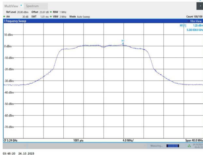
11AC20MIMO_Ant2_5240
