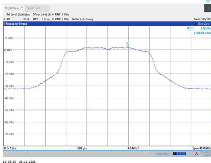
11A_Ant2_5700
