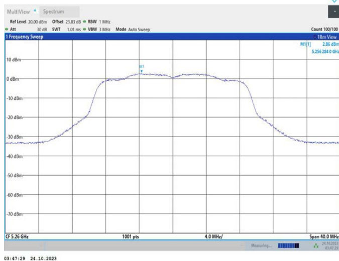
11AC20MIMO_Ant2_5260
