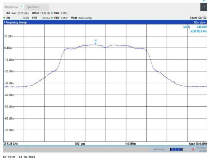
11A_Ant2_5260
