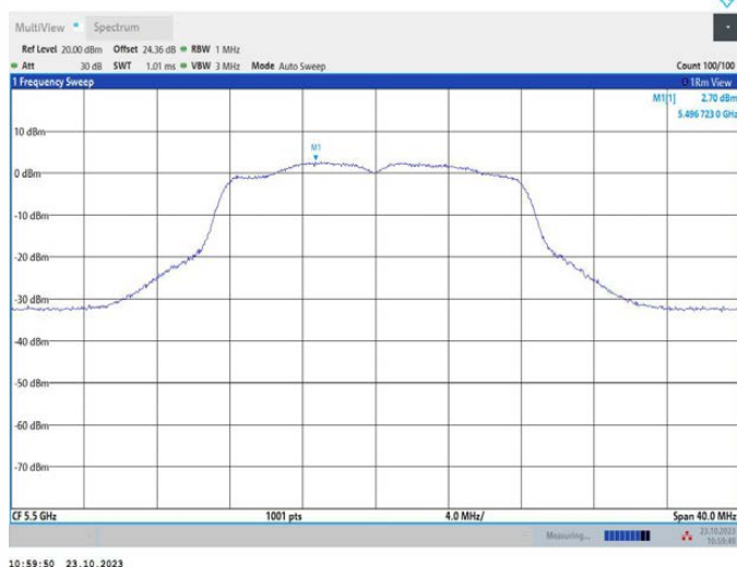
11A_Ant2_5500
