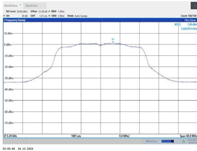
11AC20MIMO_Ant2_5240
