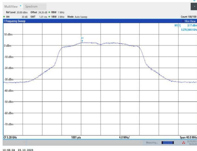
11A_Ant1_5280
