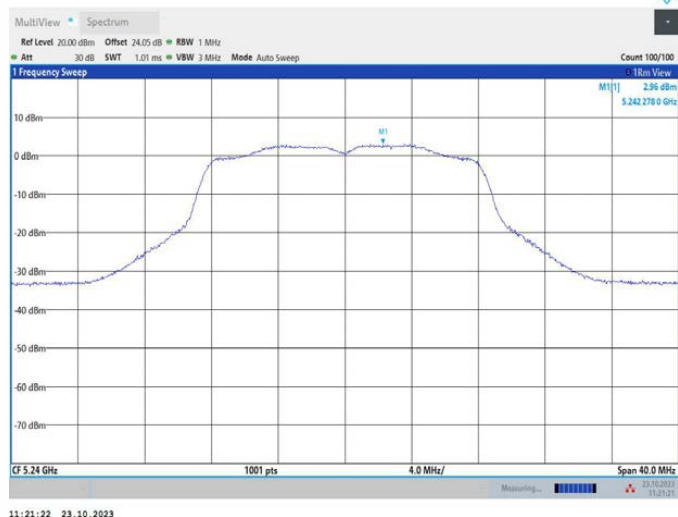
11A_Ant2_5240
