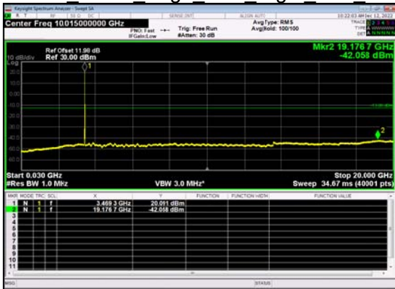
N77(20M)_DFT-s- OFDM BPSK Edge 1RB Right Low CH
