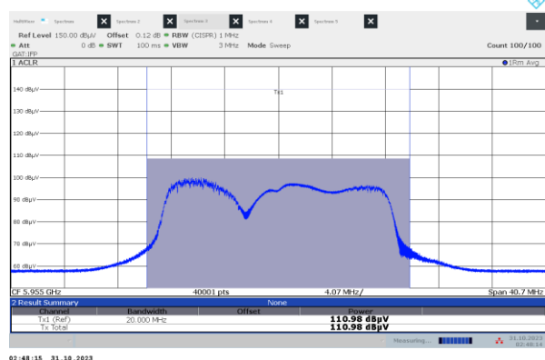
802.11a / CH 1
