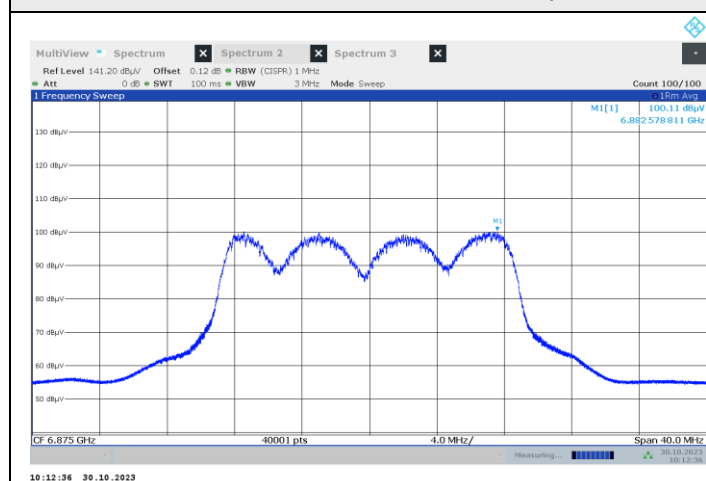
802.11a / CH 185
