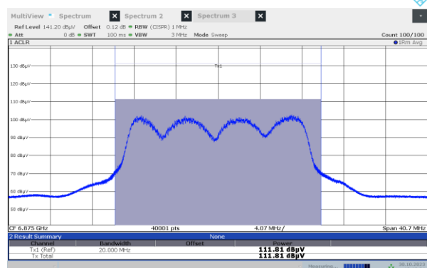
802.11a / CH 185
