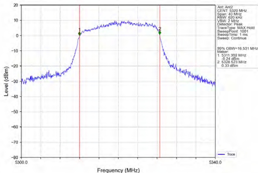
802.11a_HCH_5320MHz_Ant2_NTNV
