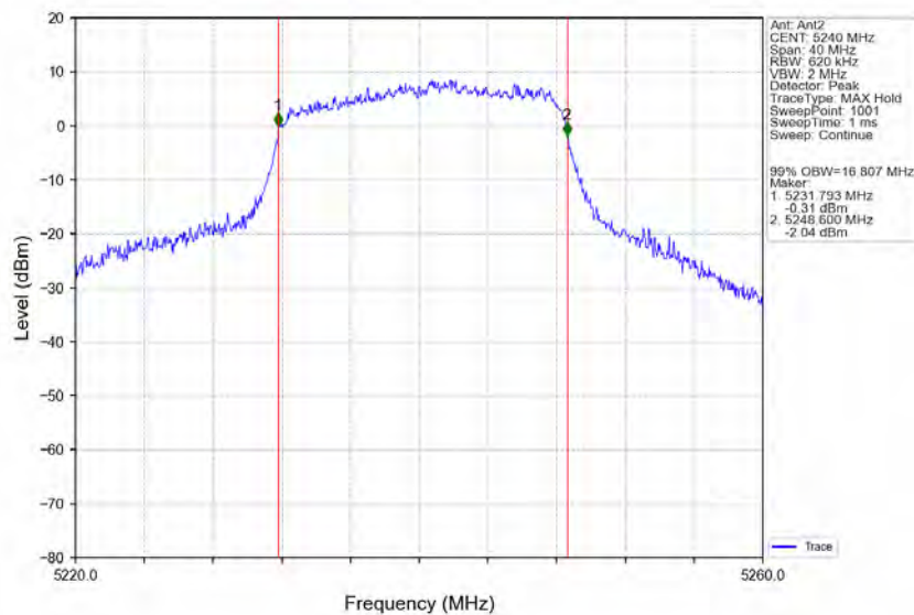
802.11a_HCH_5240MHz_Ant2_NTNV
