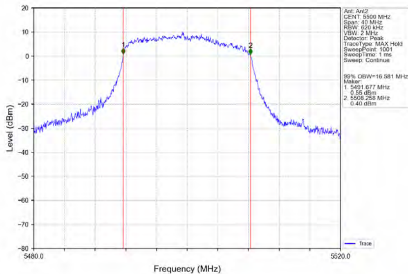
802.11a_LCH_5500MHz_Ant2_NTNV
