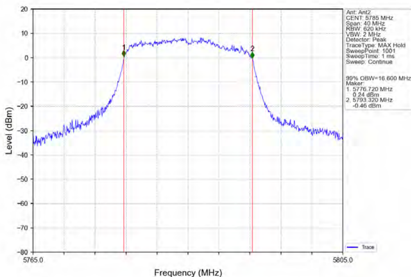
802.11a_MCH_5785MHz_Ant2_NTNV
