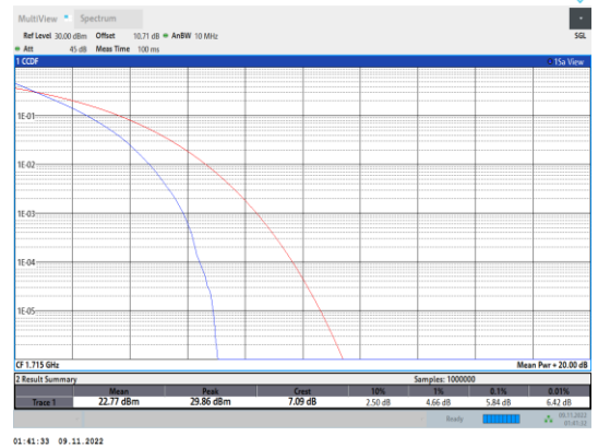
Band4-10MHz-QPSK-20000-50RB#0
