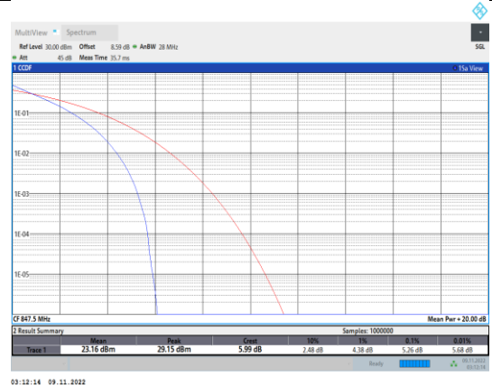
Band5-3MHz-QPSK-20635-15RB#0
