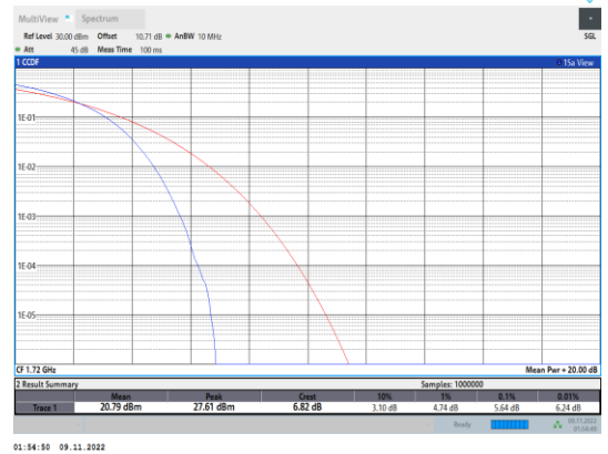
Band4-20MHz-QPSK-20050-100RB#0
