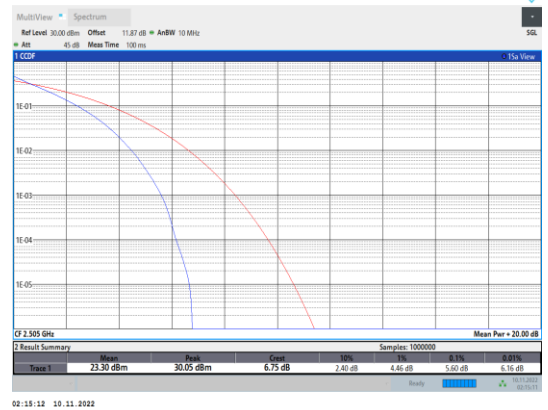
Band7-10MHz-QPSK-20800-50RB#0
