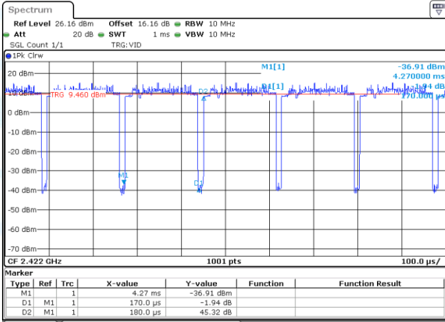
NTNV-11AX40MIMO-Ant1-2422
