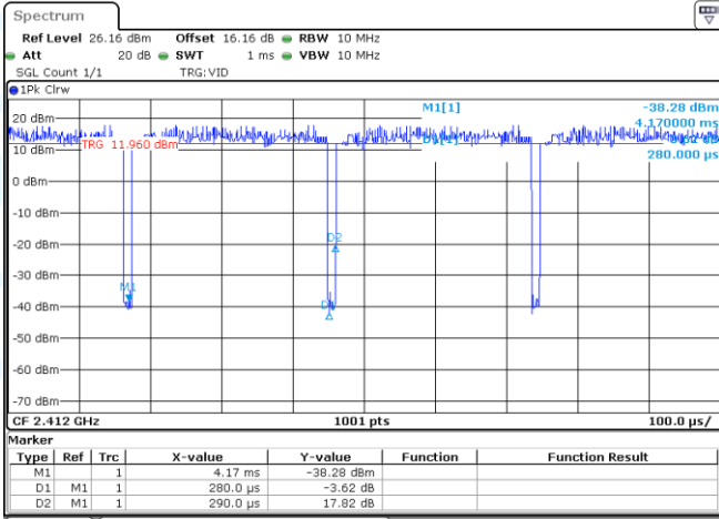
NTNV-11AX20MIMO-Ant1-2412
