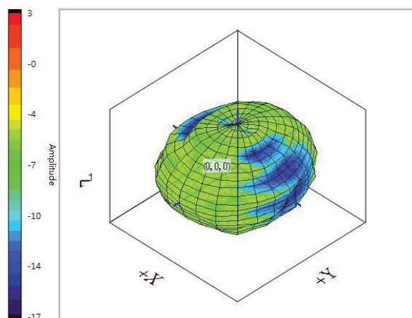
5500 MHz
