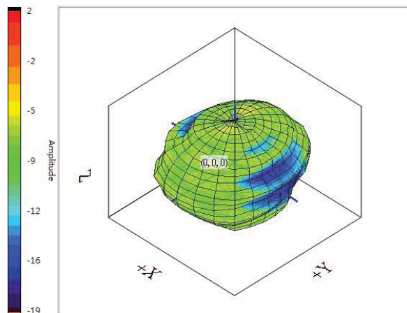
5150 MHz
