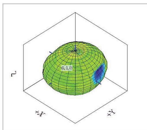
2450 MHz
