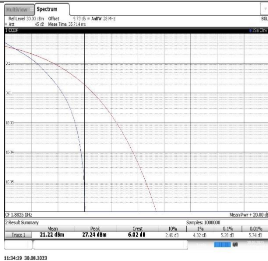
Band25-10MHz-QPSK-26365-50RB#0
