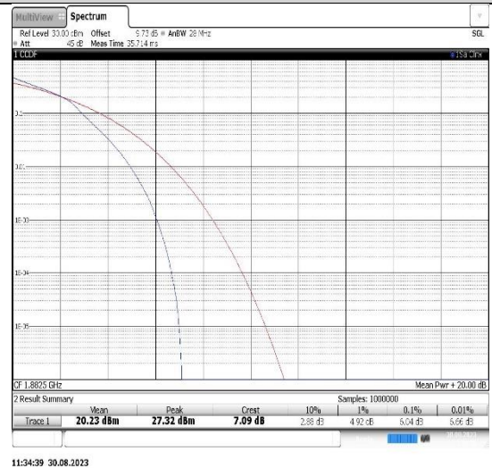
Band25-10MHz-16QAM-26365-50RB#0
