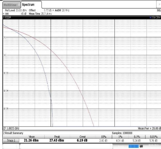
Band25-1.4MHz-QPSK-26365-6RB#0
