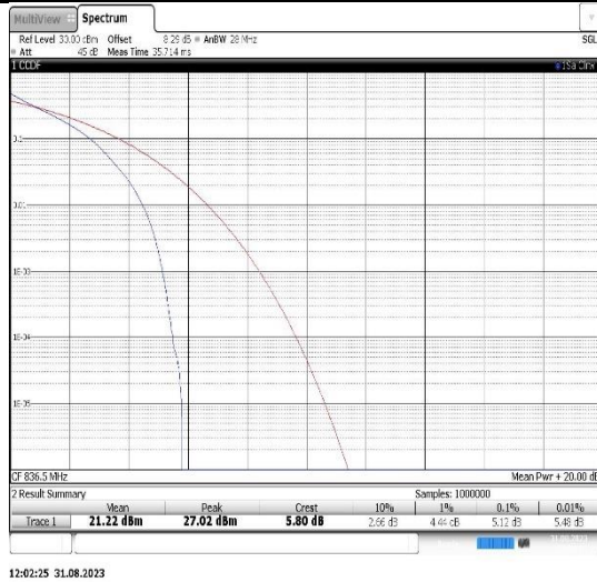
Band26(824-849)-3MHz-QPSK-26915-15RB#0
