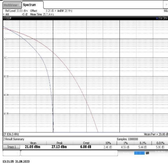
Band26(824-849)-10MHz-QPSK-26915-50RB#0
