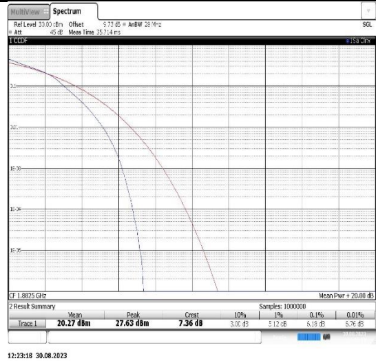
Band25-20MHz-16QAM-26365-100RB#0
