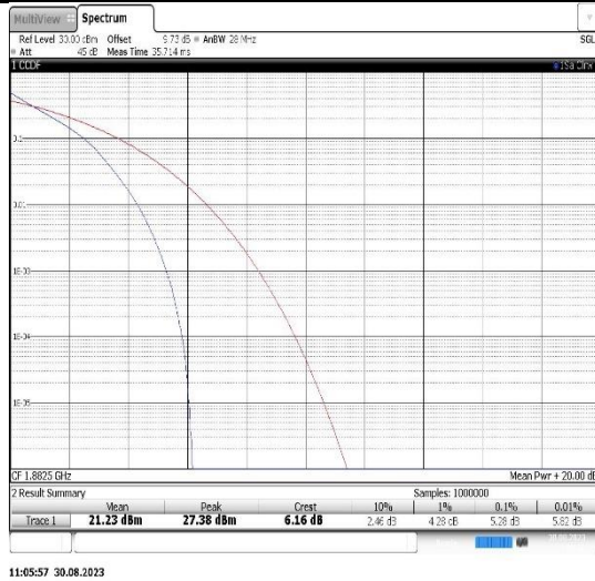
Band25-5MHz-QPSK-26365-25RB#0
