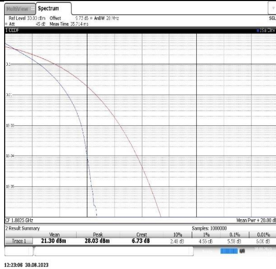
Band25-20MHz-QPSK-26365-100RB#0
