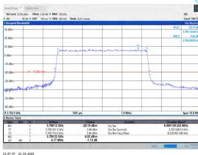
Band43-5MHz-QPSK-45090-25RB#0
