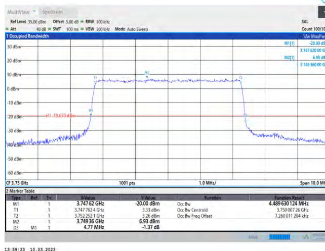
Band43-5MHz-QPSK-45090-25RB#0
