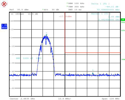
b_2462MHz_Chain 0 44.21dB
