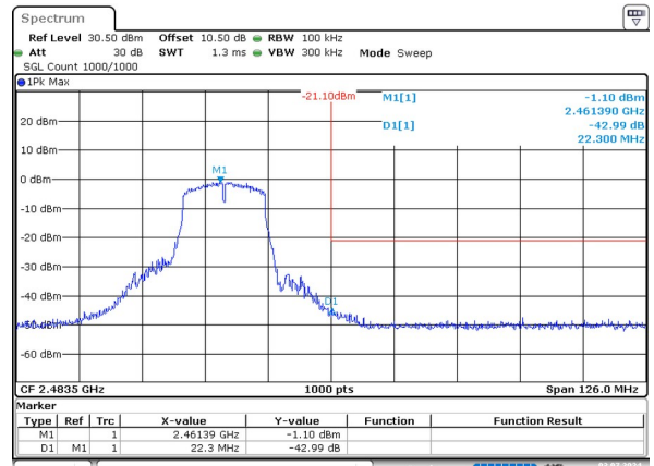
g_2462MHz_Chain 1 42.99dB
