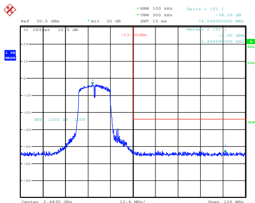
n20_2462MHz_Chain 0 38.39dB
