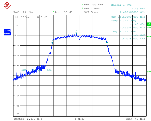
g_2412MHz_Chain 0 16.520MHz
