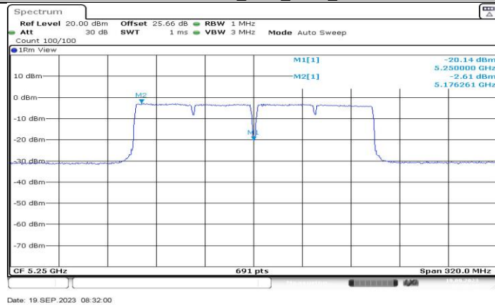
11AC160MIMO_Ant3_5250_UNII-1
