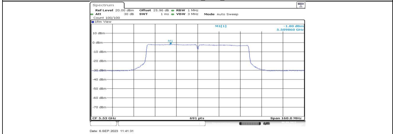
11AC80MIMO_Ant3_5530
