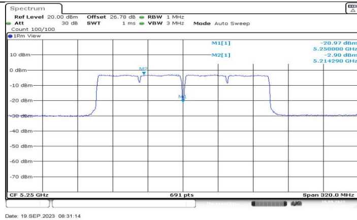
11AC160MIMO_Ant2_5250_UNII-1
