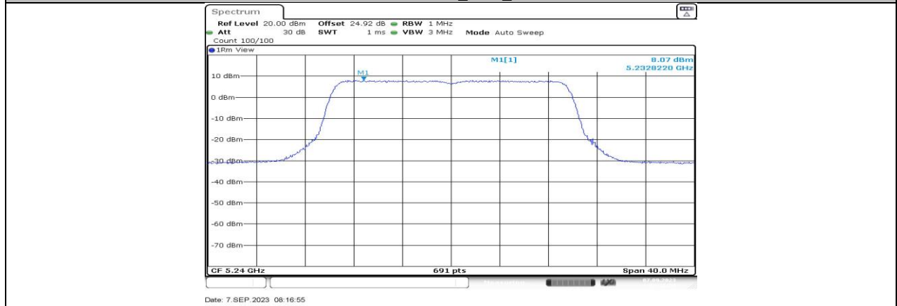
11BE20MIMO_Ant4_5240
