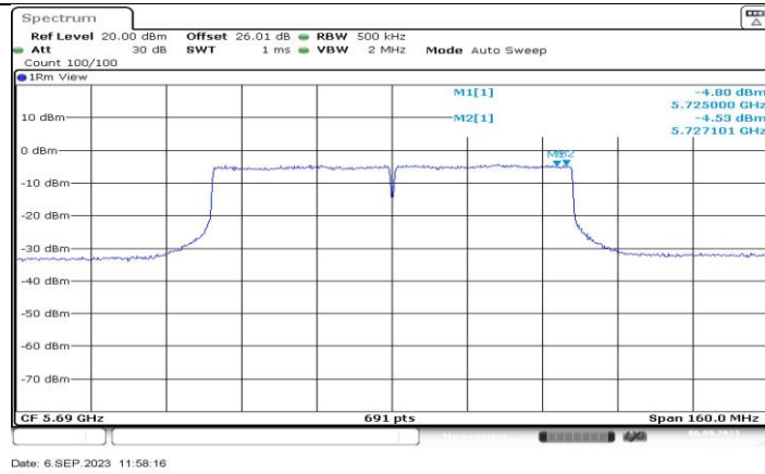
11AC80MIMO_Ant3_5690_UNII-3
