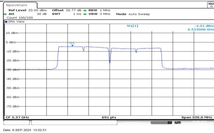
11AC160MIMO_Ant1_5570
