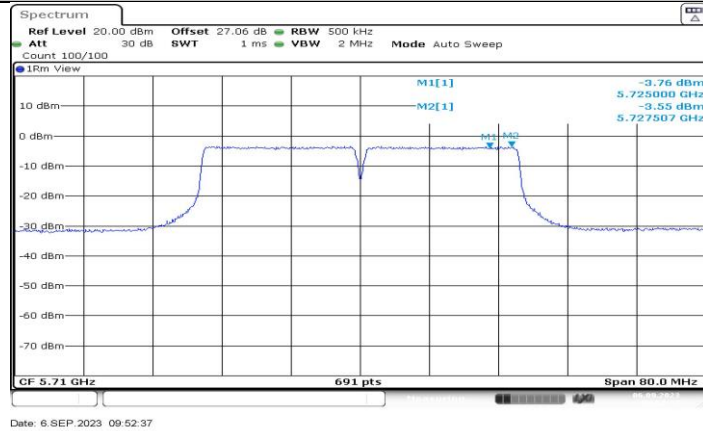
11AC40MIMO_Ant2_5710_UNII-3
