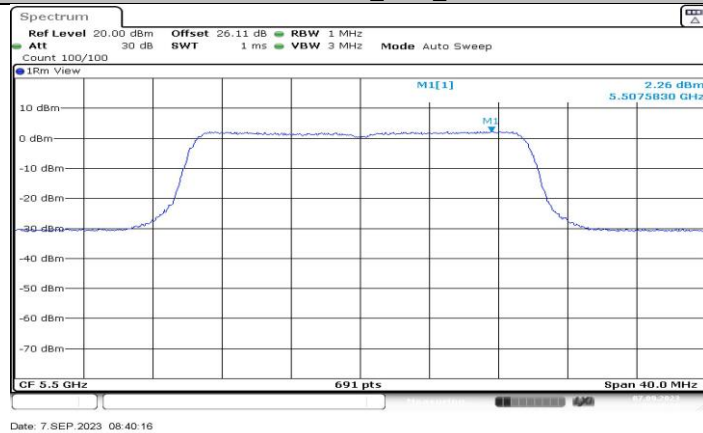
11BE20MIMO_Ant2_5500
