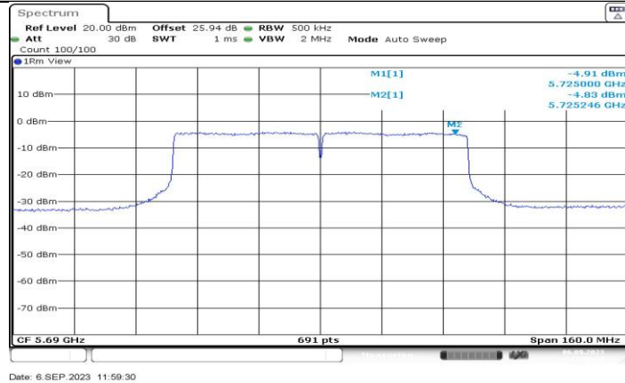
11AC80MIMO_Ant4_5690_UNII-3
