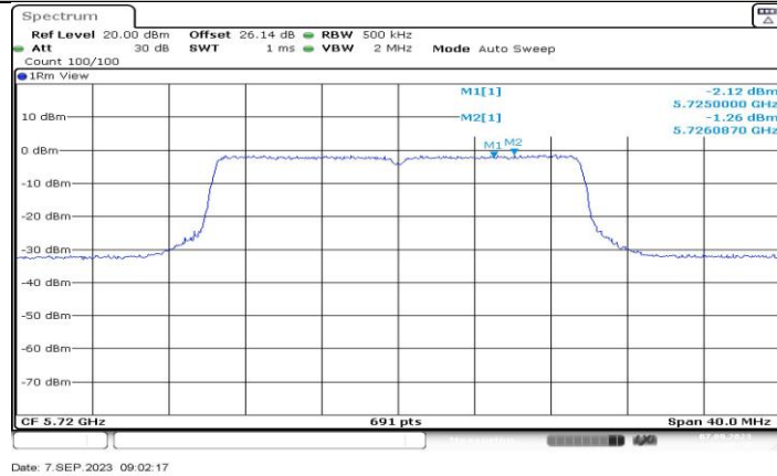
11BE20MIMO_Ant1_5720_UNII-3
