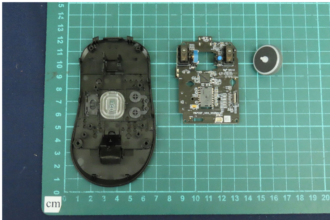
(9) EUT Photo
