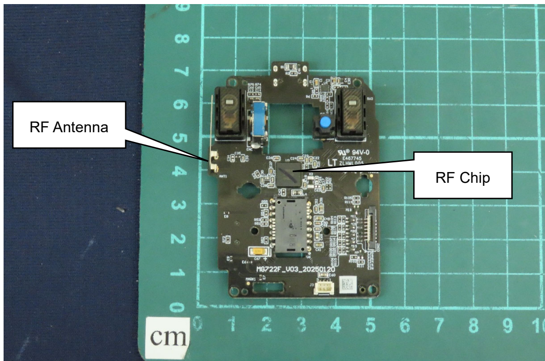
(10) EUT Photo
