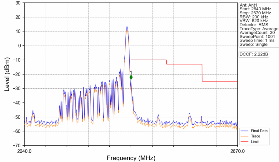
Band41_10MHz_QPSK_HCH_2650MHz_RB_1_49_NTNV
