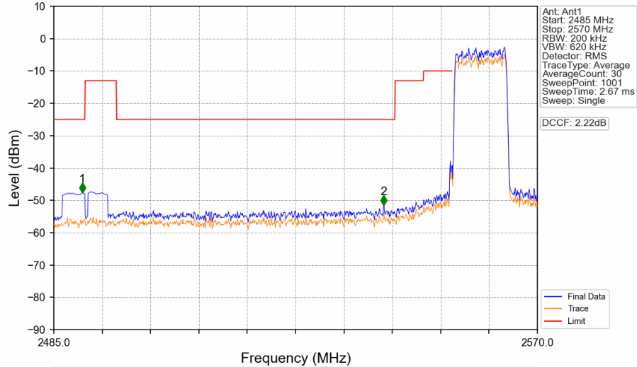
Band41_10MHz_16QAM_LCH_2560MHz_RB_50_0_NTNV
