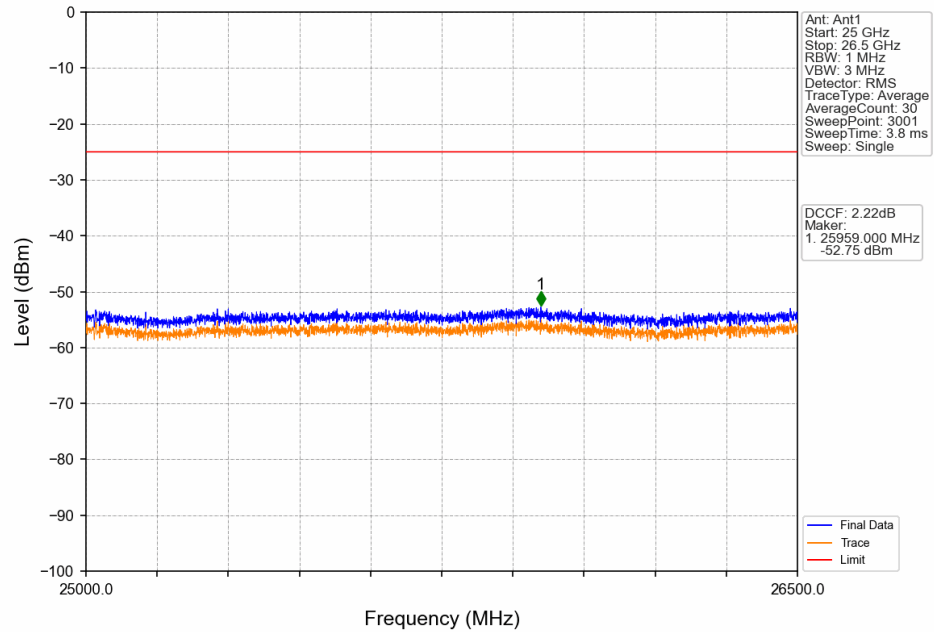
Band41_10MHz_QPSK_MCH_2605MHz_RB_1_0_NTNV
