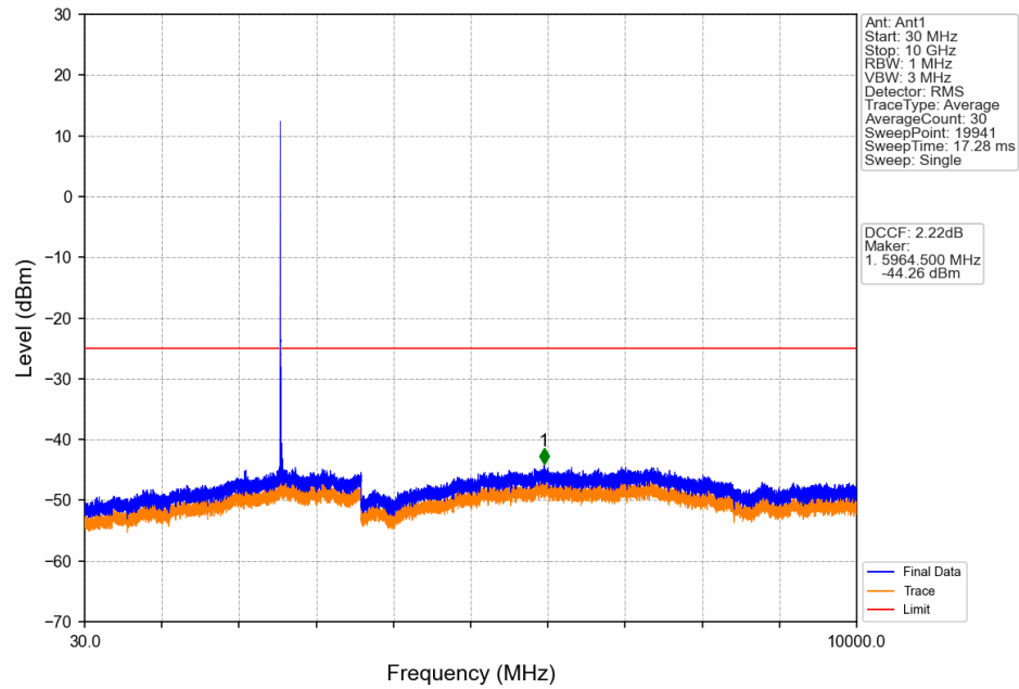
Band41_10MHz_16QAM_LCH_2560MHz_RB_1_0_NTNV
