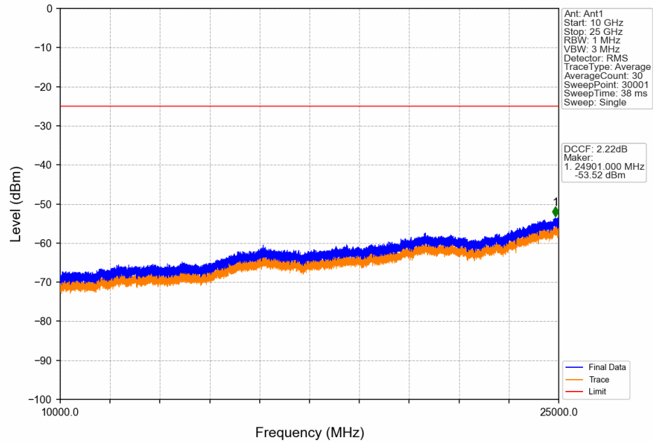
Band41_10MHz_QPSK_HCH_2650MHz_RB_1_0_NTNV
