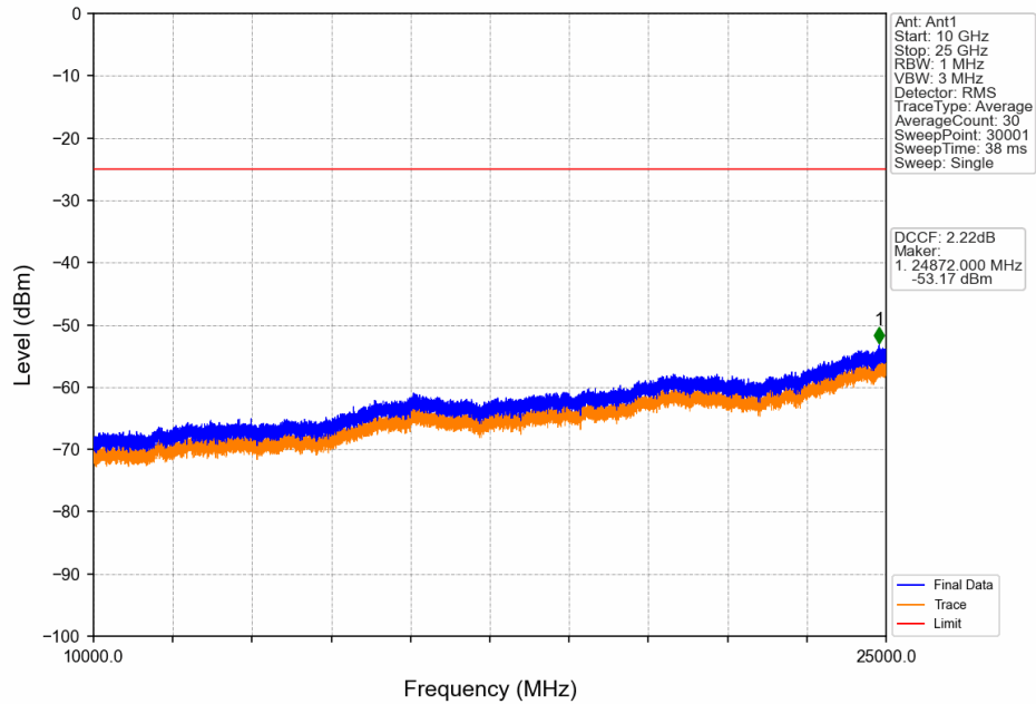
Band41_15MHz_QPSK_HCH_2647.5MHz_RB_1_0_NTNV
