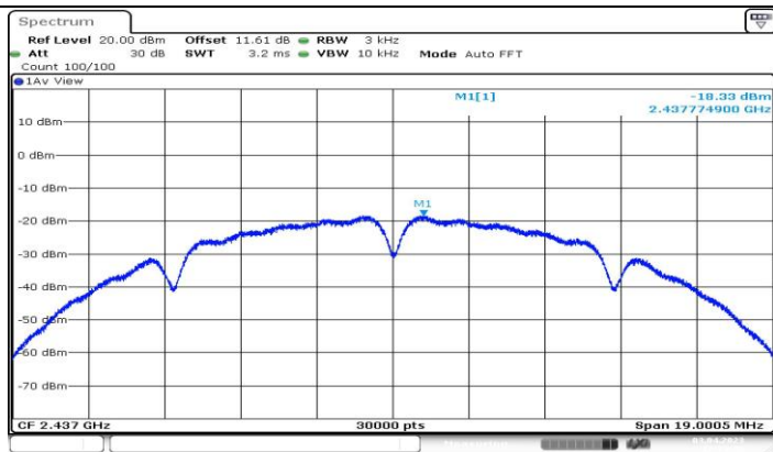
11B_Ant1_2437
