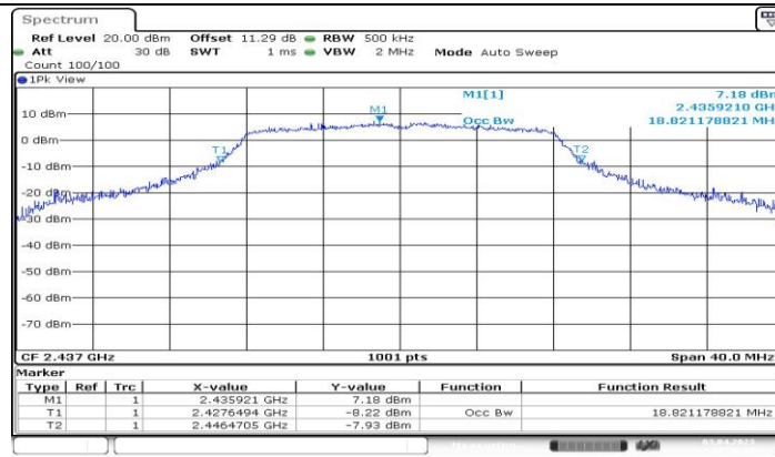
11G_Ant1_2437
