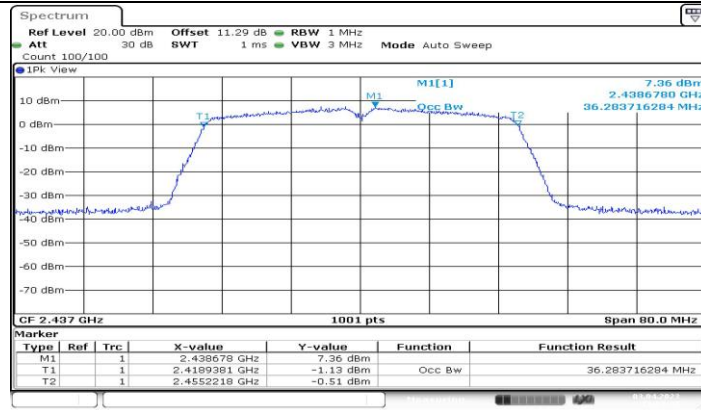
11N40MIMO_Ant1_2437
