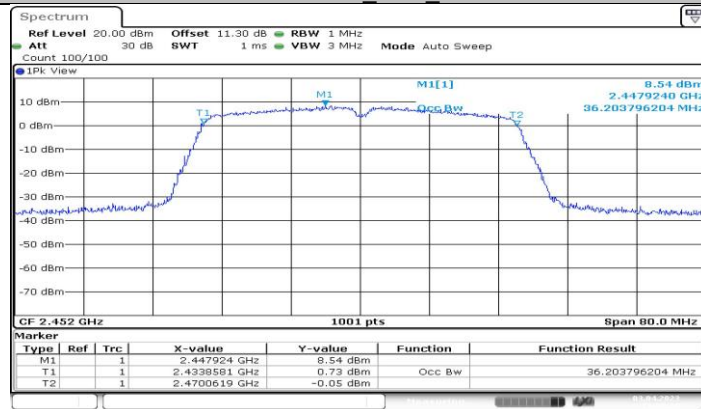
11N40MIMO_Ant0_2452
