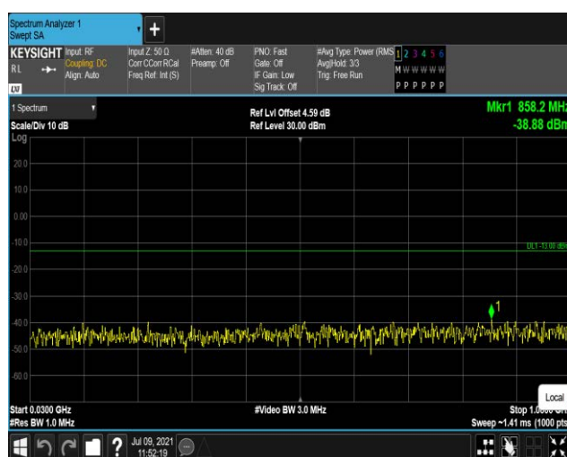
Band2-1.4MHz-QPSK-19193:30~1000MHz
