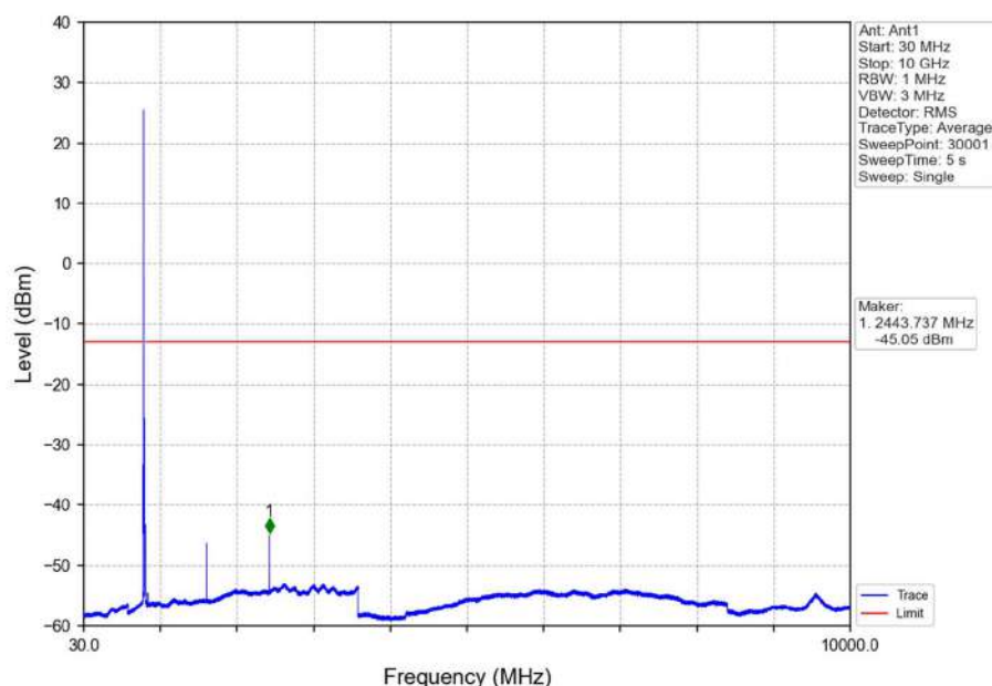
Band26a_10MHz_QPSK_MCH_819MHz_RB_1_0_NTNV
