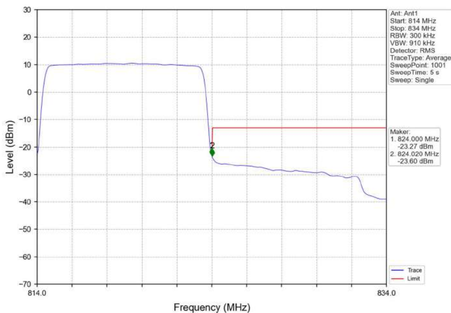
Band26a 10MHz QPSK HCH 819MHz RB 50 0 NTN
