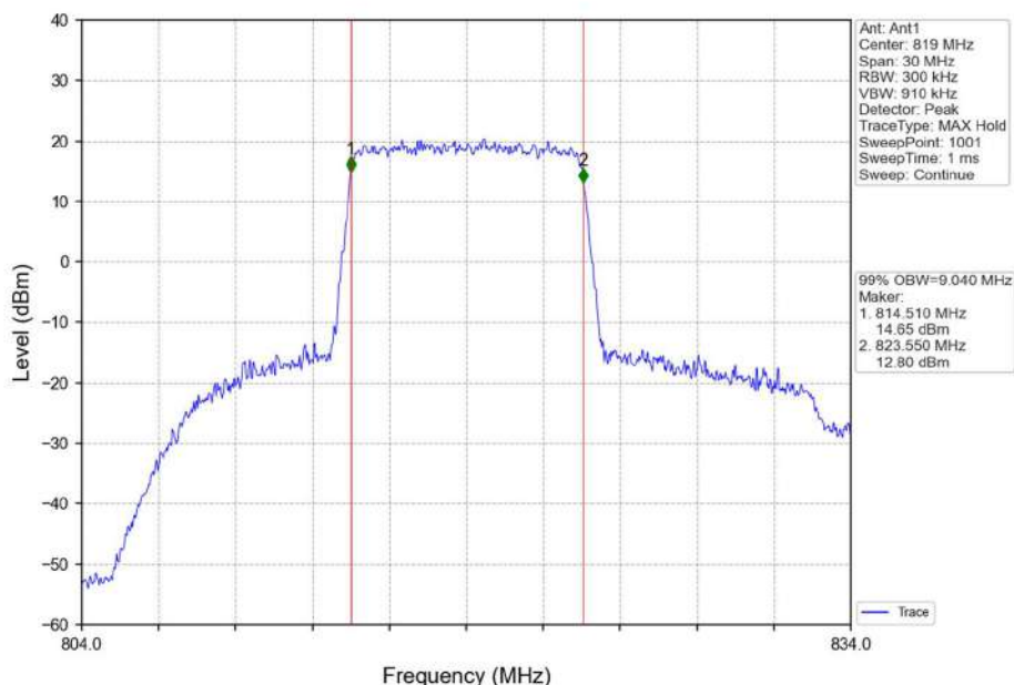
Band26a_10MHz_QPSK_MCH_819MHz_RB_50_0_NTNV
