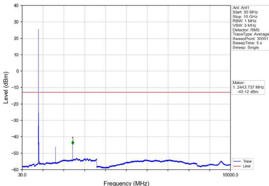
Band26a_10MHz_QPSK_LCH_819MHz_RB_1_0_NTNV
