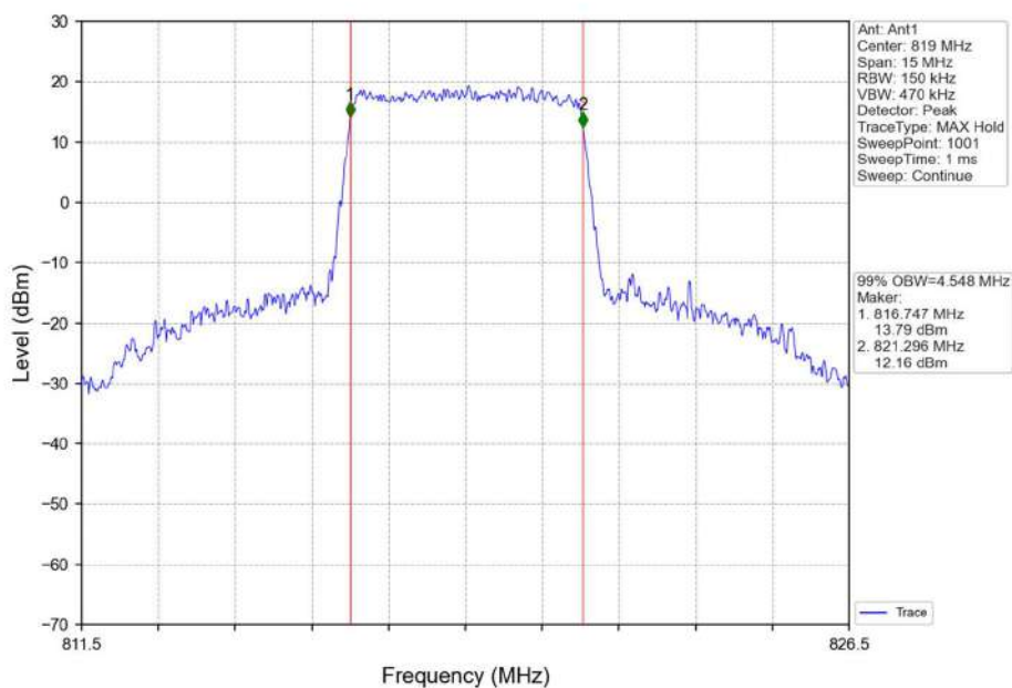
Band26a 5MHz 16QAM MCH 819MHz RB 25 0 NTNV
