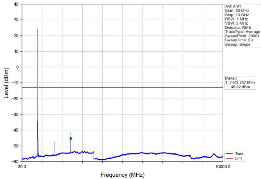
Band26a 10MHz 16QAM MCH 819MHz RB 1 0 NTNV
