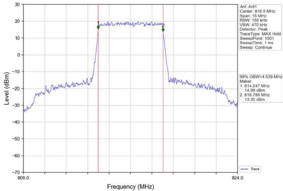
Band26a 5MHz QPSK LCH 816.5MHz RB 25 0 NTN
