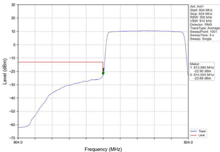
Band26a 10MHz QPSK LCH 819MHz RB 50 0 NTN
