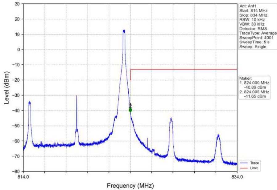
Band26a 10MHz 16QAM HCH 819MHz RB 1 49 NTNV
