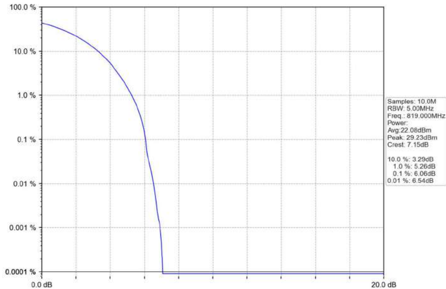
Band26a 10MHz QPSK HCH 819MHz RB 50 0 NTN
