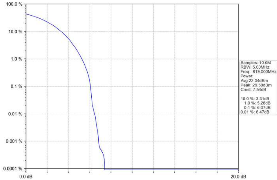
Band26a_10MHz_QPSK_MCH_819MHz_RB_50_0_NTNV
