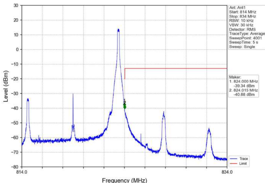
Band26a_10MHz_QPSK_HCH_819MHz_RB_1_49_NTNV
