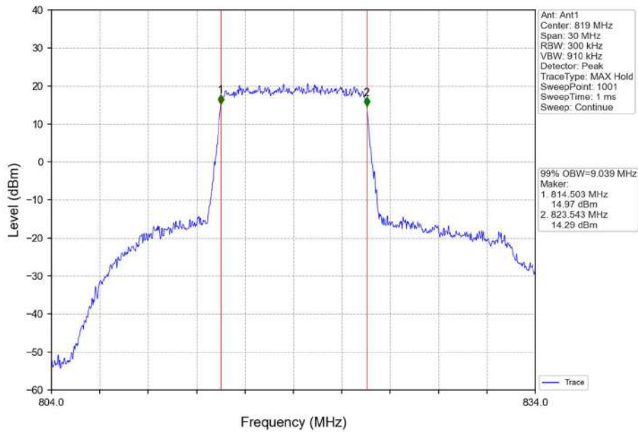
Band26a 10MHz QPSK HCH 819MHz RB 50 0 NTN
