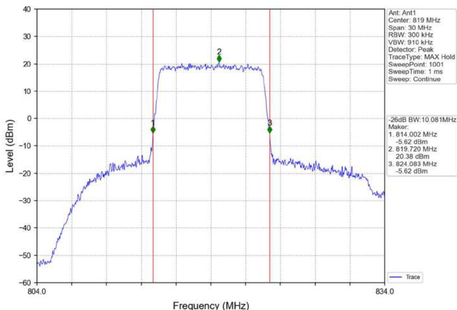
Band26a_10MHz_QPSK_MCH_819MHz_RB_50_0_NTNV
