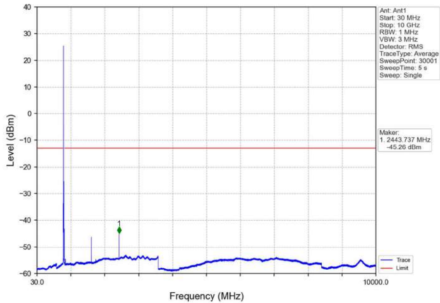
Band26a 10MHz QPSK HCH 819MHz RB 1 0 NTNV
