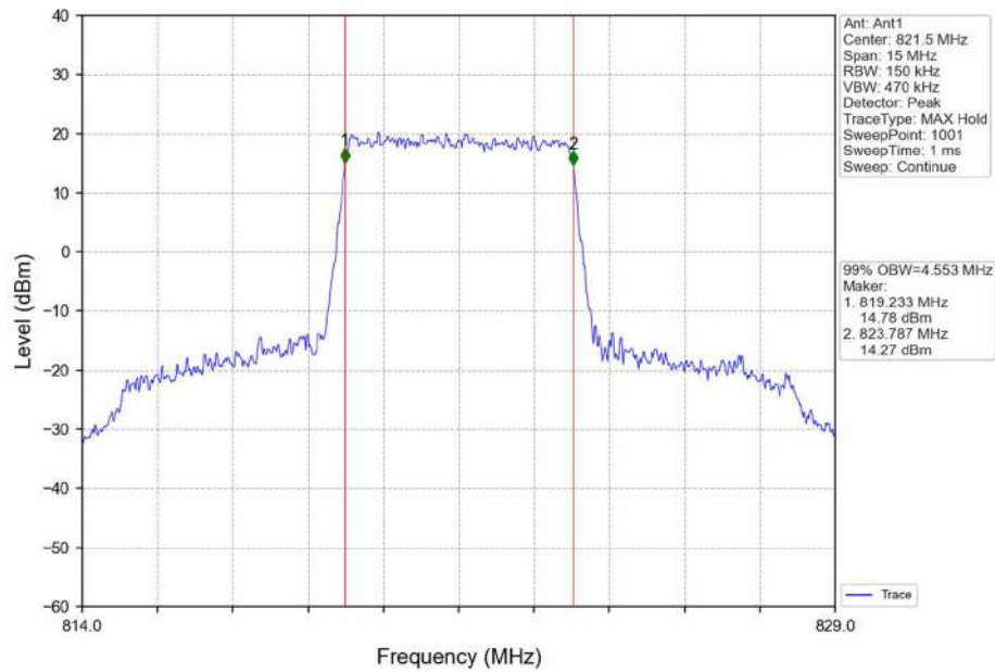
Band26a 5MHz QPSK HCH 821.5MHz RB 25 0 NTN
