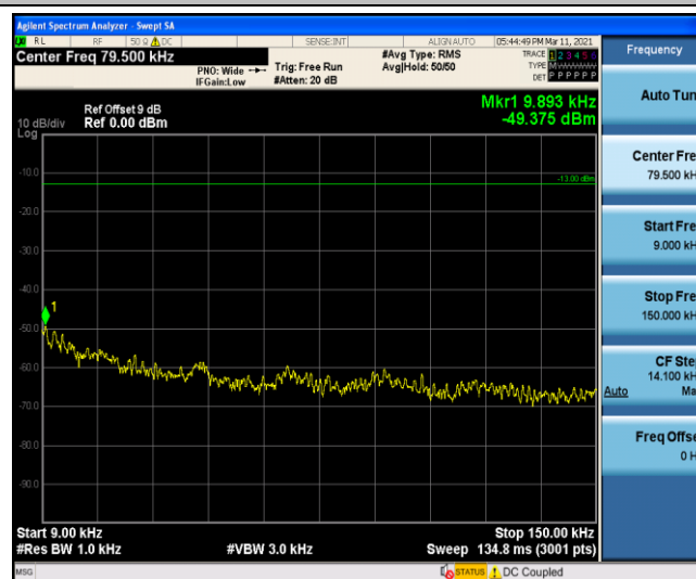
Band 71_10MHz_QPSK_133172_1RB#0
