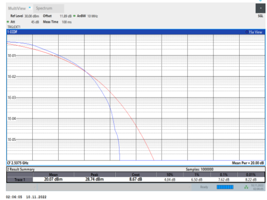
Band41-5MHz-QPSK-40065-25RB#0
