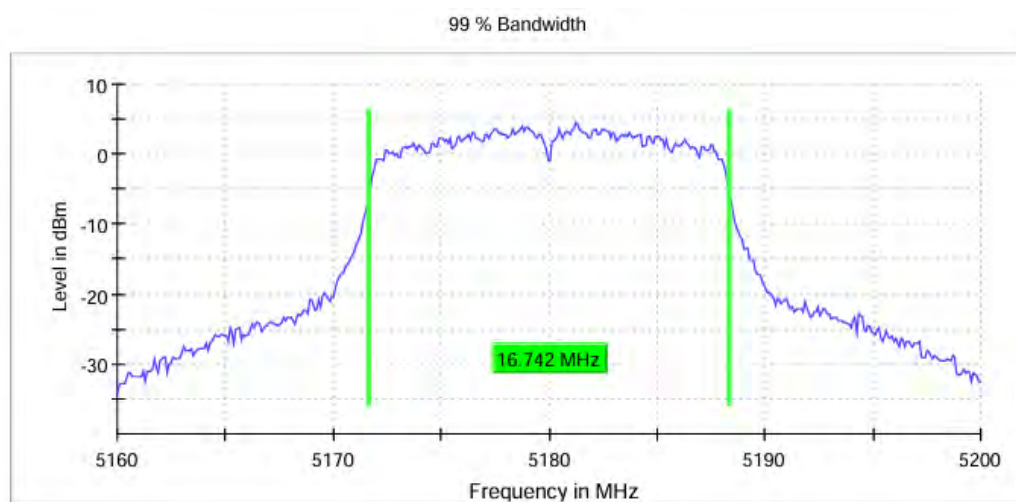
11A_Ant0_5180
