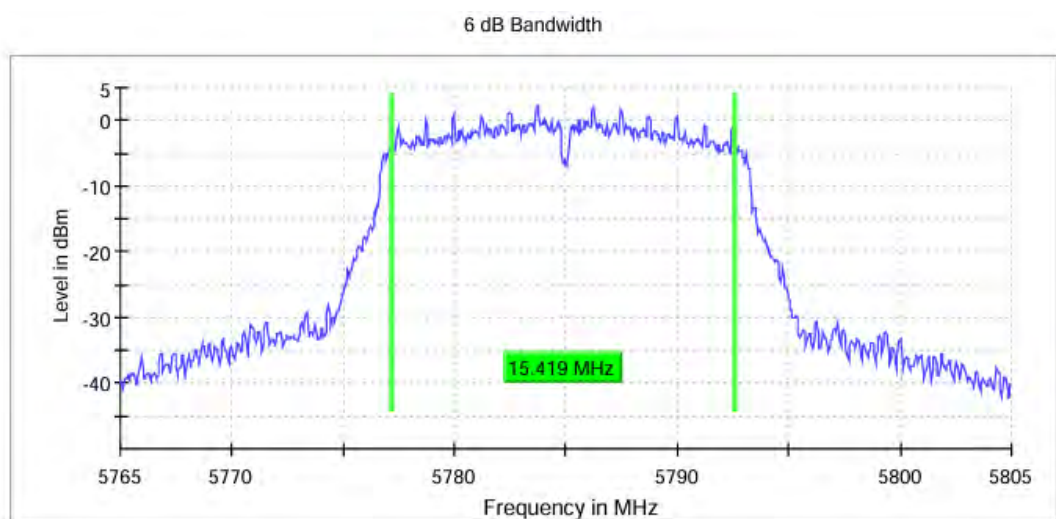
11A_Ant0_5785
