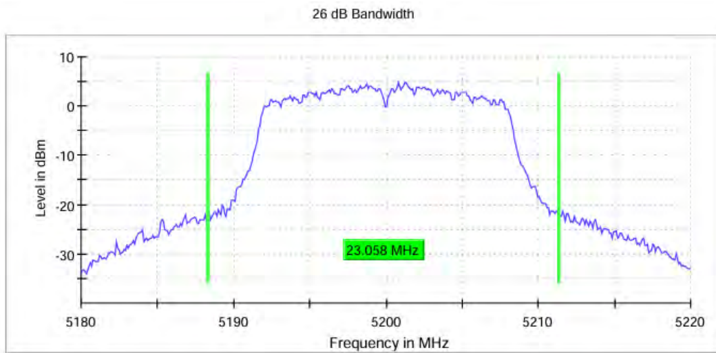
11A_Ant0_5200
