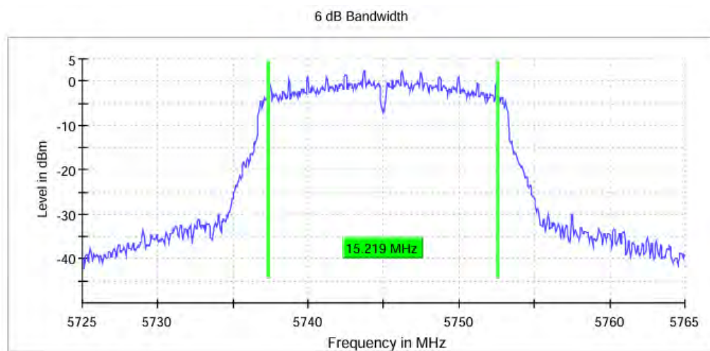
11A_Ant0_5745
