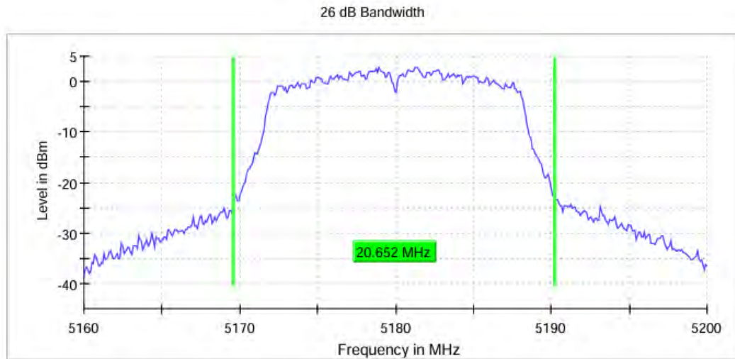
11A_Ant0_5180
