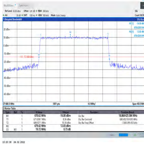
1-N71-PC3-15-20-M-7-CP-16QAM-Outer_Ful I-106@0-Ant1-18.868-19.720-≤20-PASS
